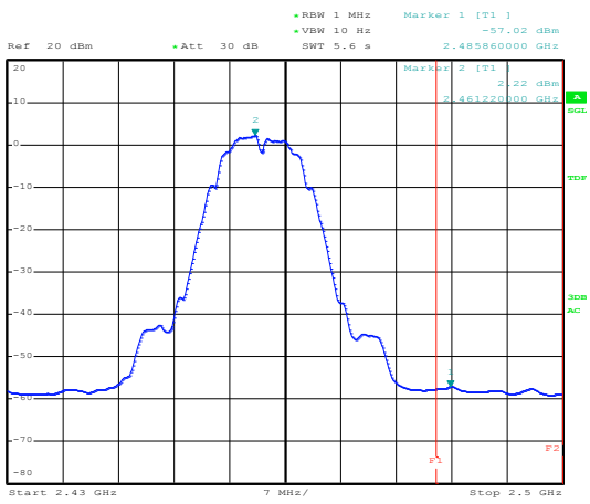
Antenna 0 IEEE 802.11b
