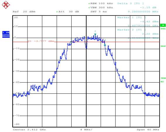
Antenna 1 IEEE 802.11b
