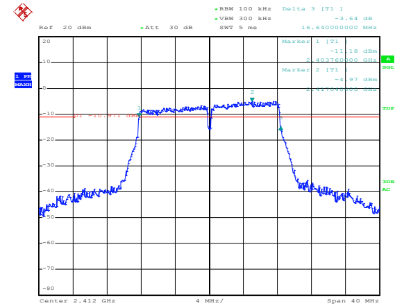
Antenna 1 IEEE 802.11g
