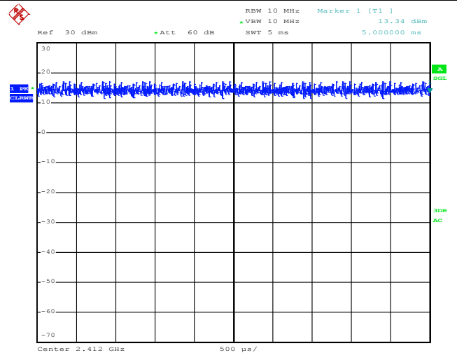
IEEE 802.11g
