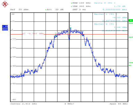
Antenna 0 IEEE 802.11b
