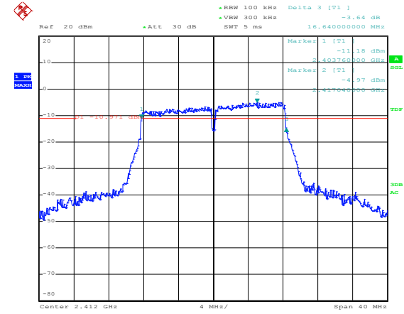
Antenna 0 IEEE 802.11g
