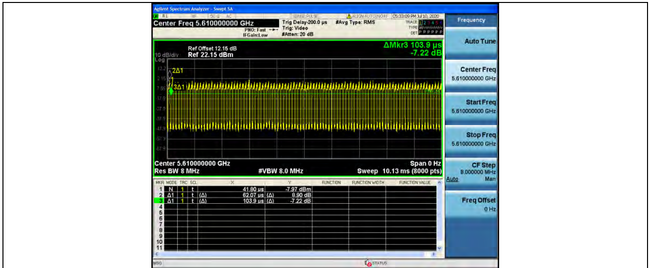
11AC80MIMO_Ant2_5610
