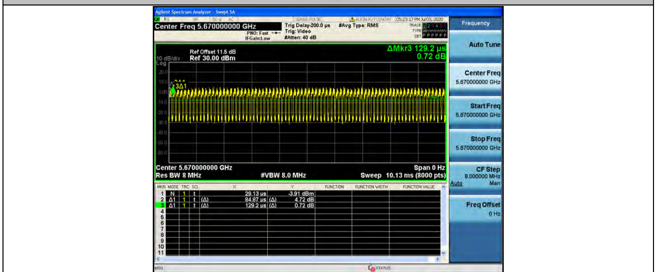
11AC40MIMO_Ant2_5670
