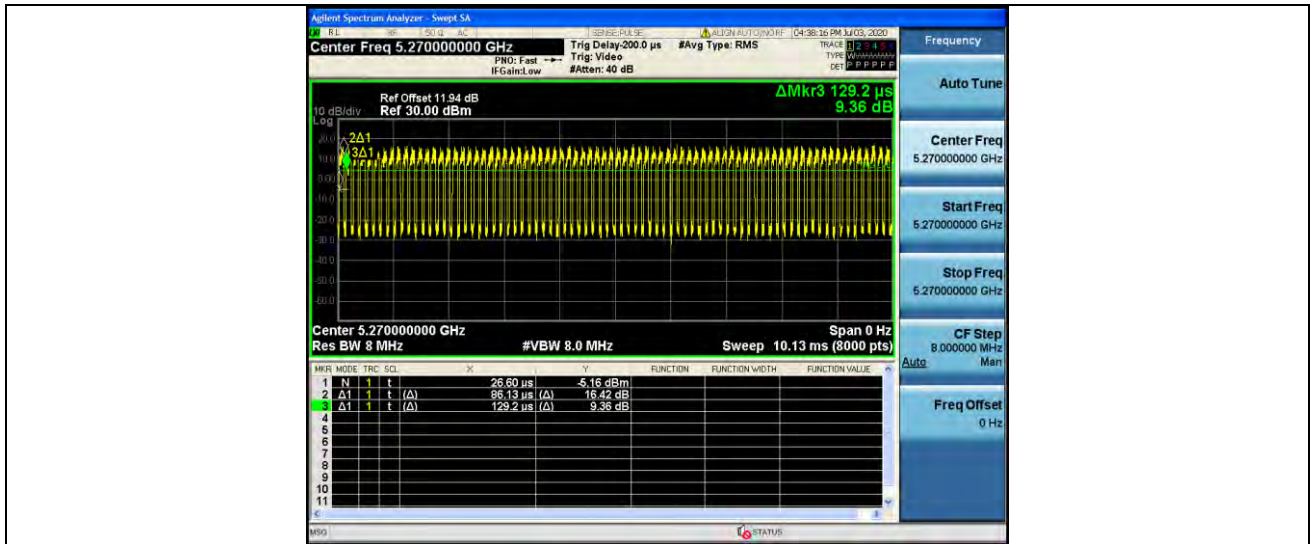
11AC40MIMO_Ant2_5270
