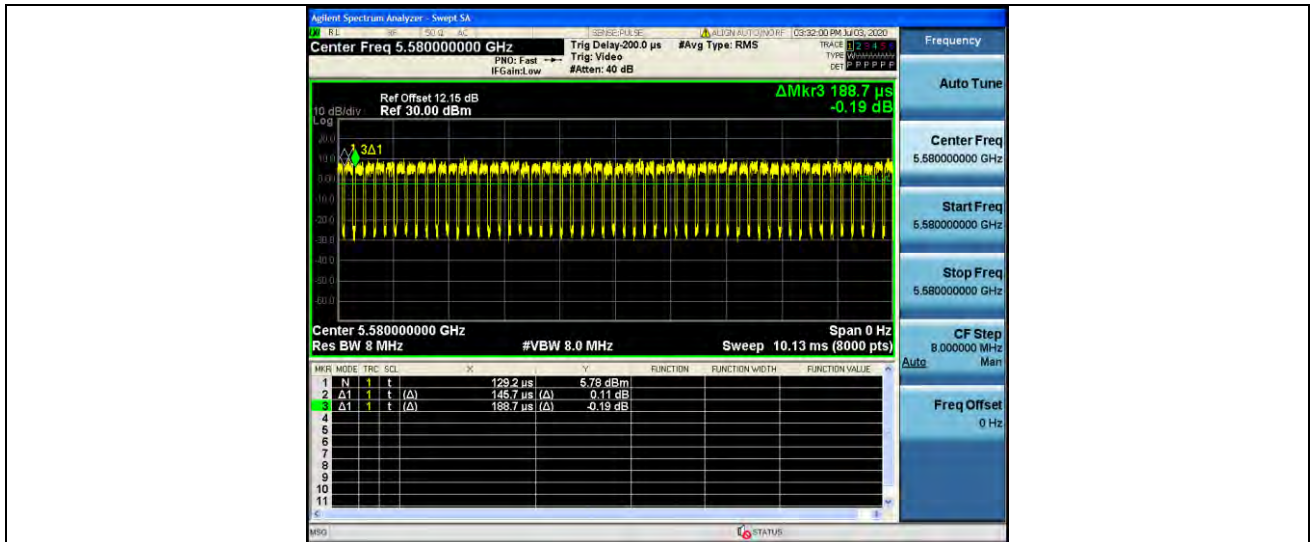
11AC20MIMO_Ant2_5580
