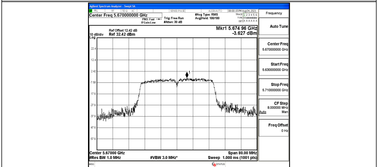
11N40MIMO_Ant2_5670
