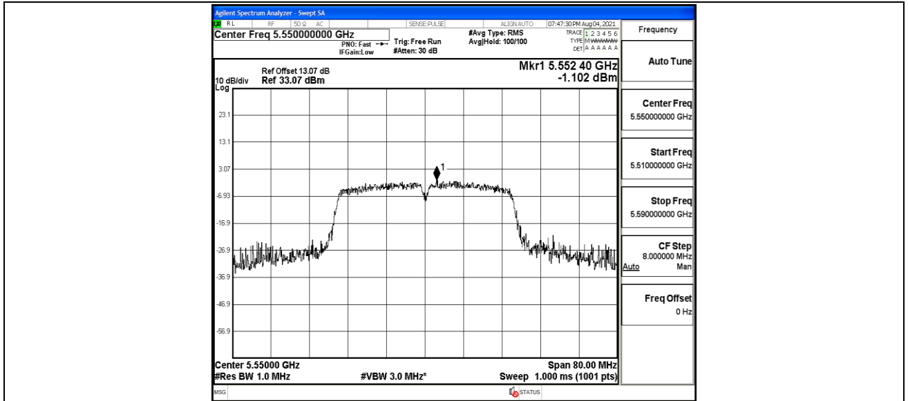
11N40MIMO_Ant2_5550
