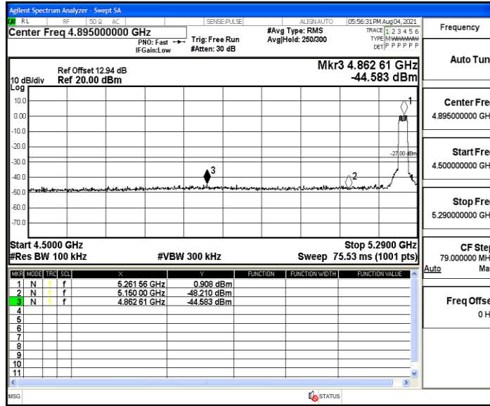
111N20MIMO_Ant2_Low_5260
