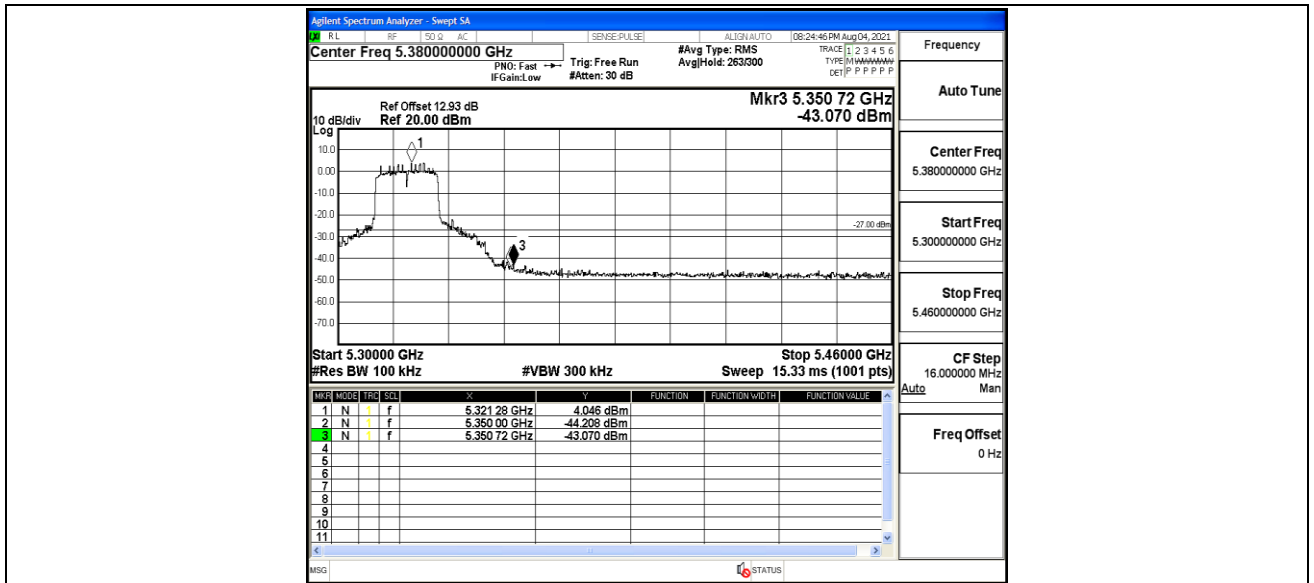
11AC20MIMO_Ant1_Low_5500
