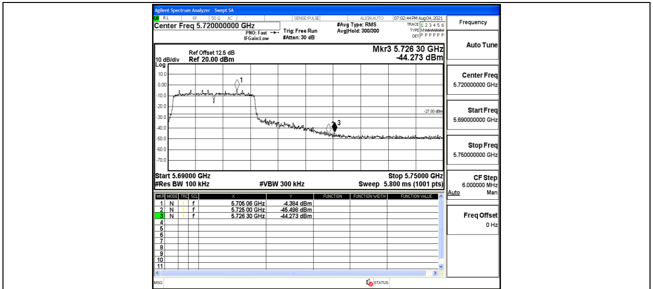
111N20MIMO_Ant2_High_5700
