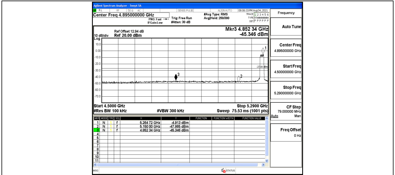
11AC20MIMO_Ant2_Low_5260
