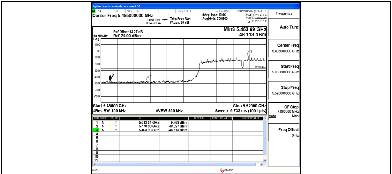
11AC40MIMO_Ant2_Low_5510
