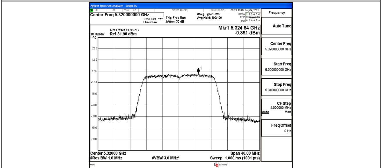
11AC20MIMO_Ant2_5320
