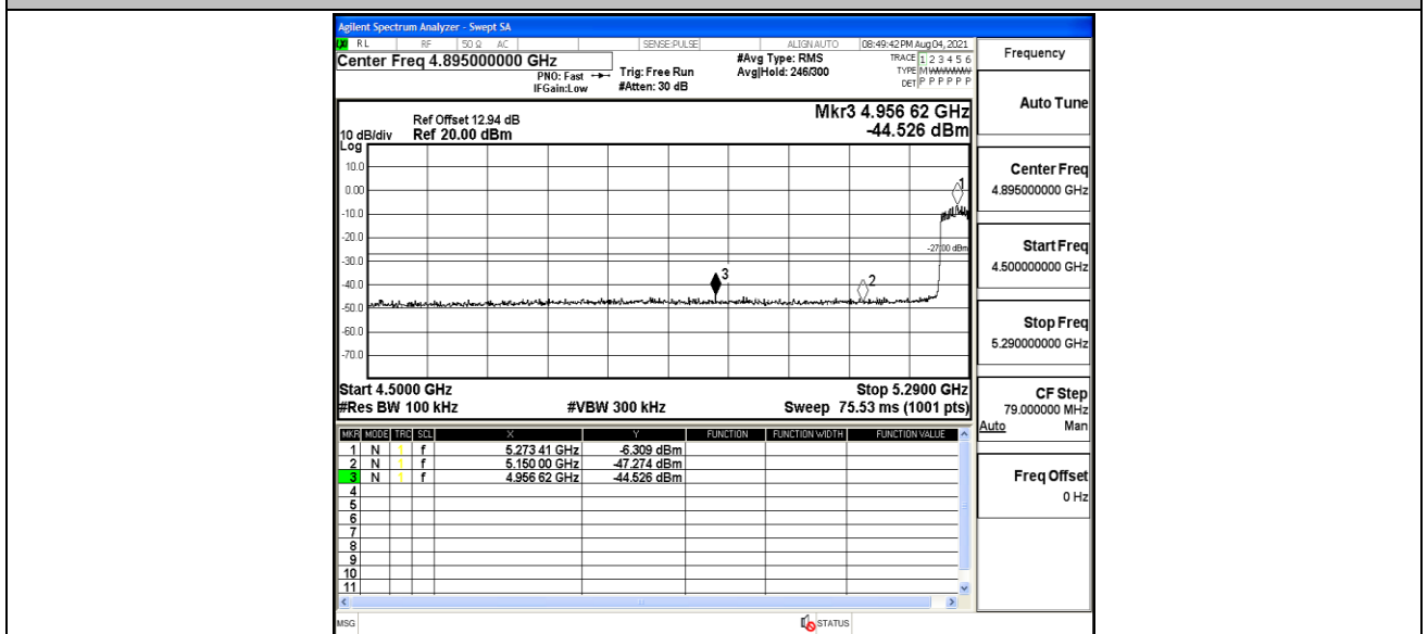
11AC40MIMO_Ant2_Low_5270
