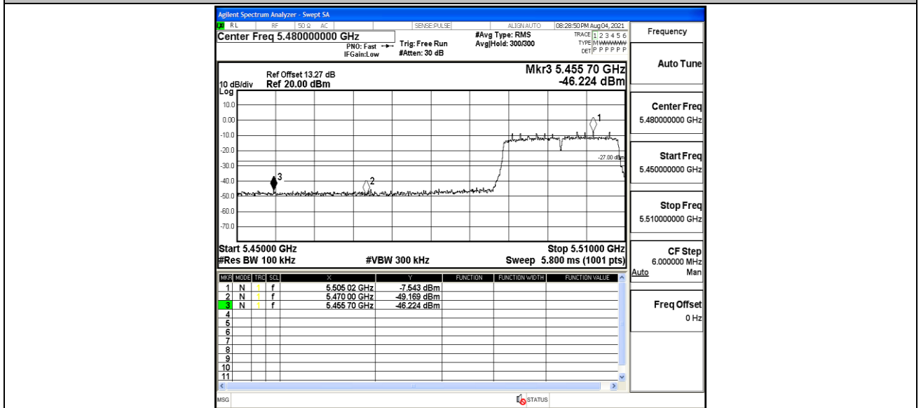
11AC20MIMO_Ant2_Low_5500
