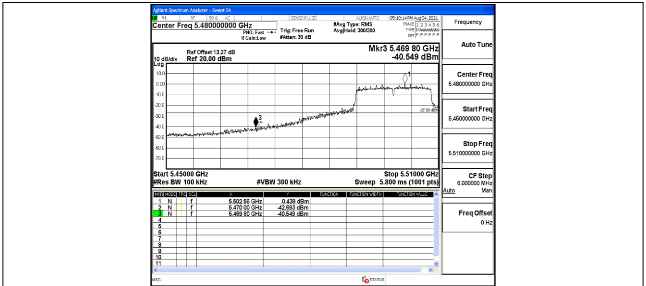
11A_Ant2_Low_5500
