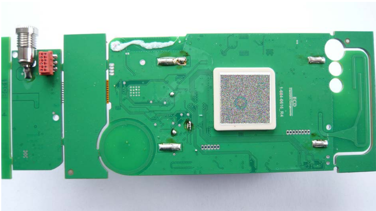
EUT Bottom:
