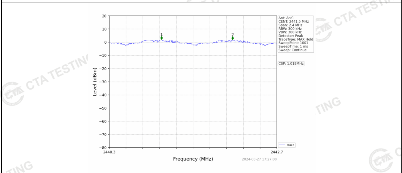
\pi/4 DQPSK
