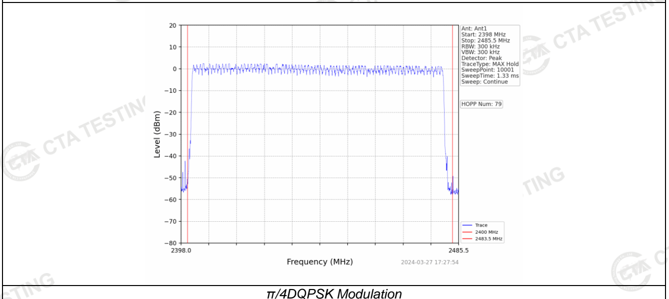
\pi/4 DQPSK Modulation
