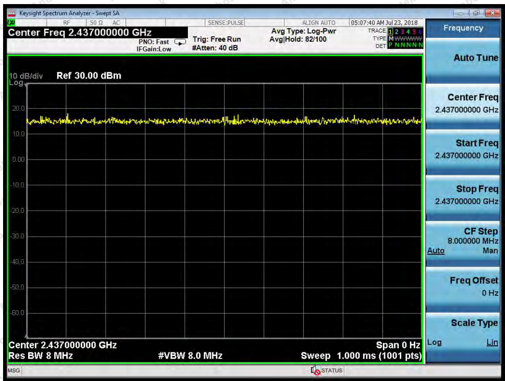
802.11n(HT20) mode
