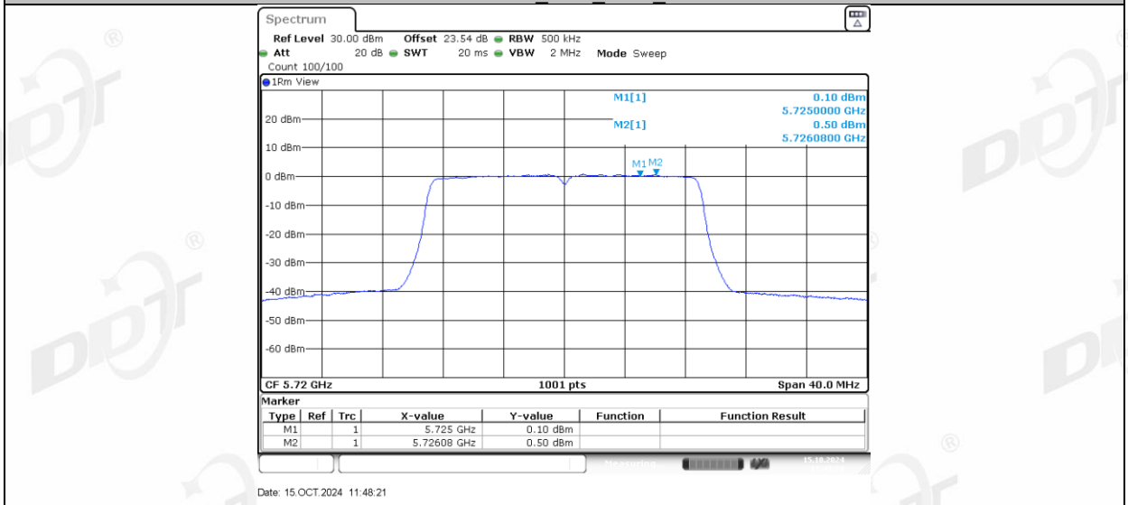
11AC20MIMO_Ant2_5720_UNII-3
