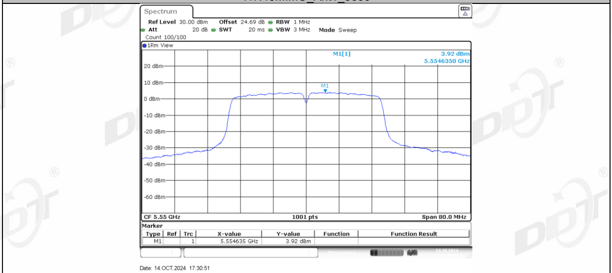
11N40MIMO_Ant2_5550
