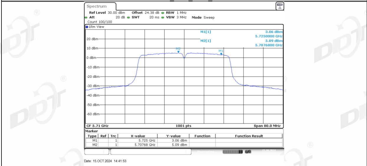
11N40MIMO_Ant1_5710_UNII-3
