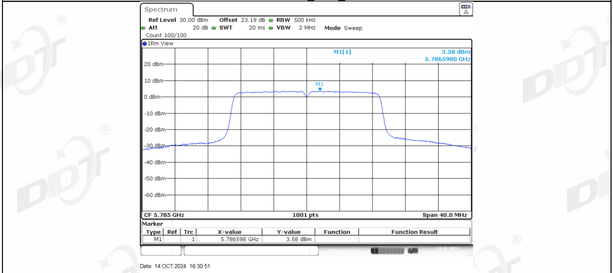
11N20MIMO_Ant2_5785
