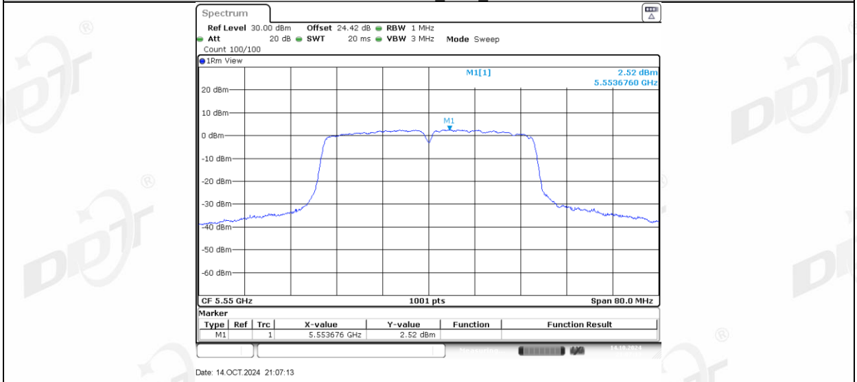
11AC40MIMO_Ant2_5550
