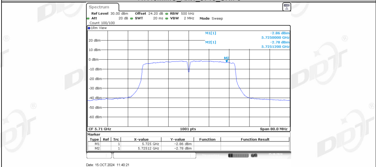
11N40MIMO_Ant2_5710_UNII-3
