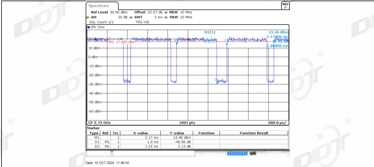
11AC20MIMO_Ant2_5720
