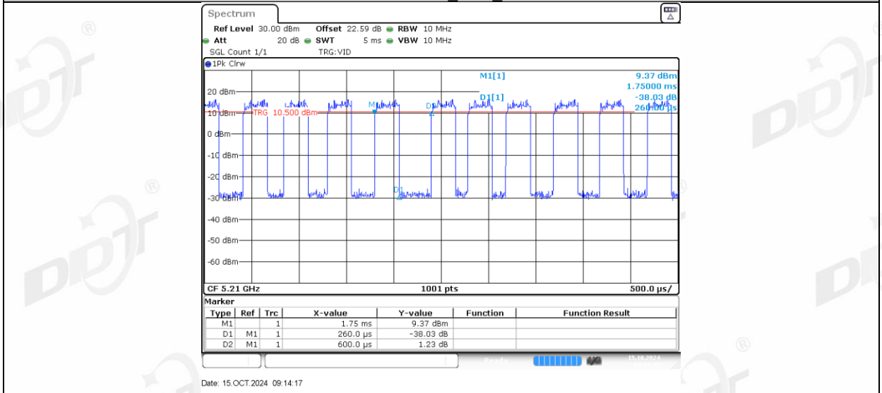
11AC80MIMO_Ant2_5210
