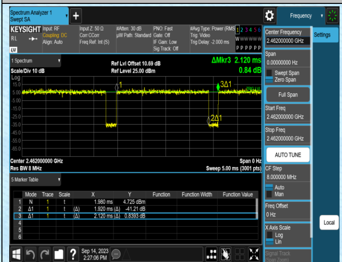
NTNV-11N20MIMO-Ant1-2462
