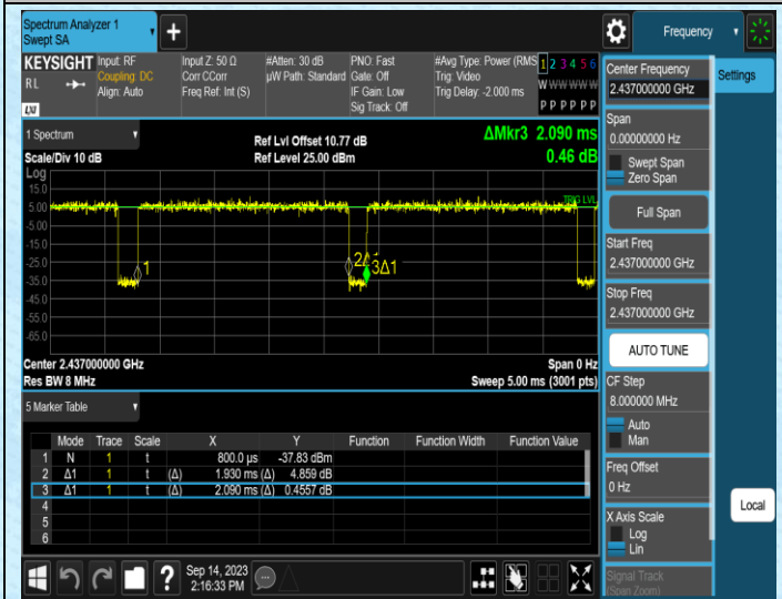
NTNV-11N20MIMO-Ant1-2437
