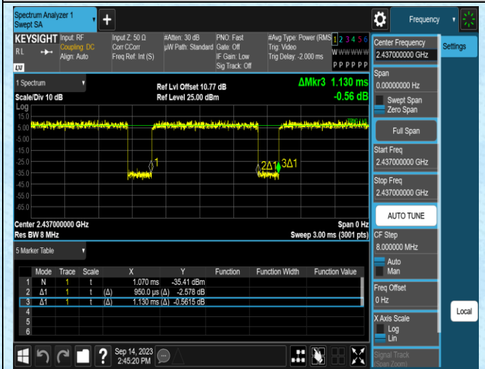
NTNV-11N40MIMO-Ant1-2437
