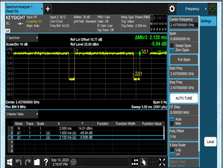
NTNV-11N20MIMO-Ant2-2437
