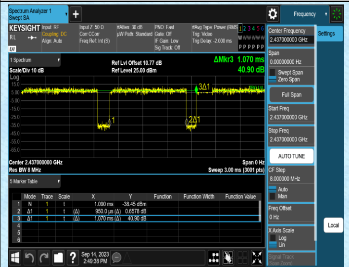
NTNV-11N40MIMO-Ant2-2437
