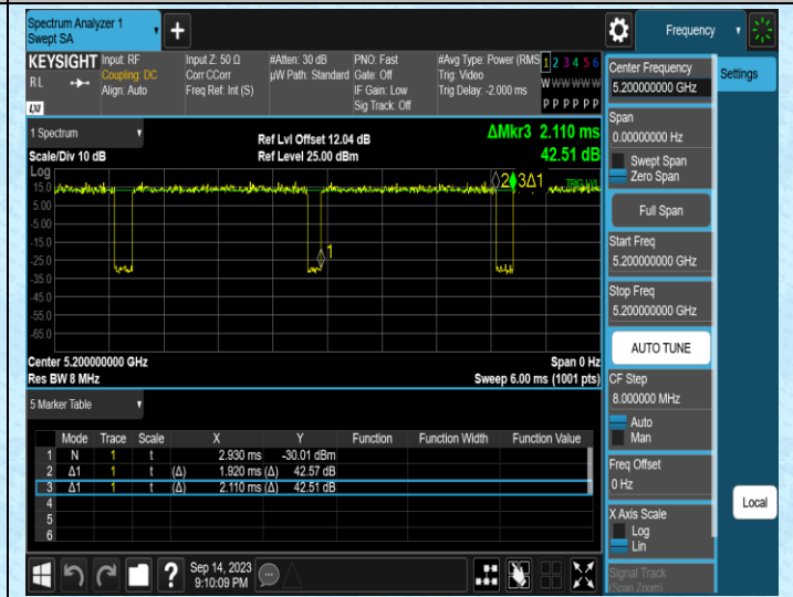
NTNV-11N20MIMO-Ant2-5200
