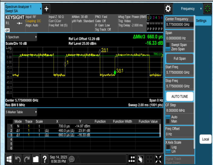
NTNV-11AC80SISO-Ant2-5775
