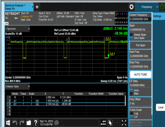
NTNV-11AC20MIMO-Ant1-5200
