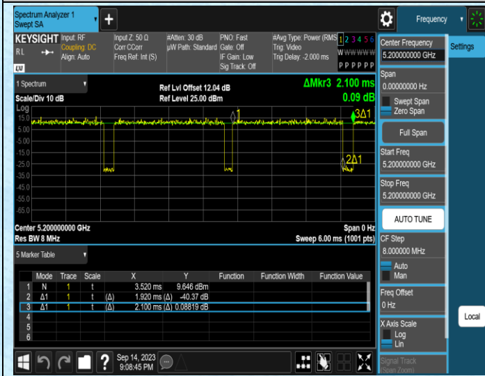
NTNV-11N20MIMO-Ant1-5200
