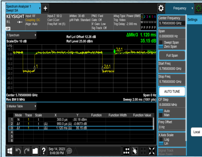
NTNV-11N40MIMO-Ant1-5795
