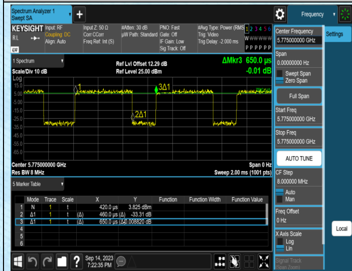
NTNV-11AC80SISO-Ant1-5775
