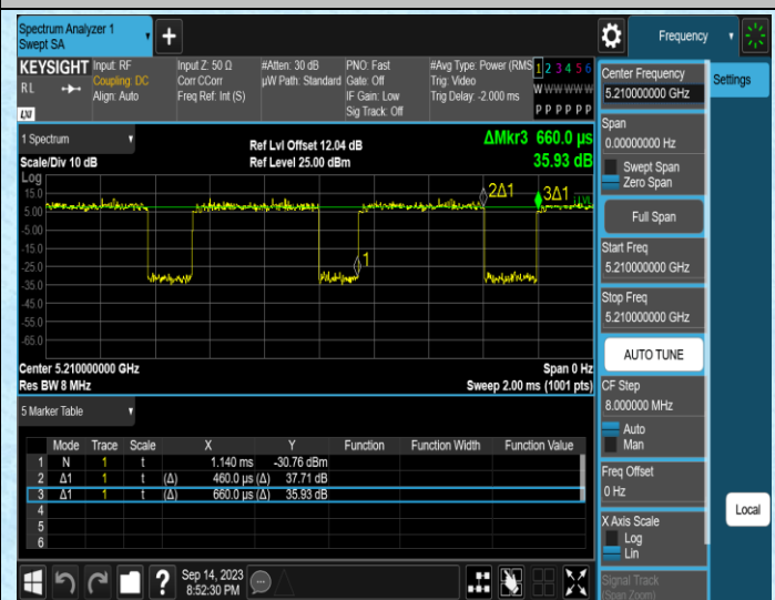
NTNV-11AC80SISO-Ant2-5210
