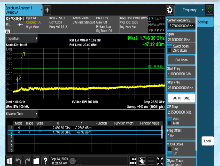
11B-Ant2-2462-1000~26500
