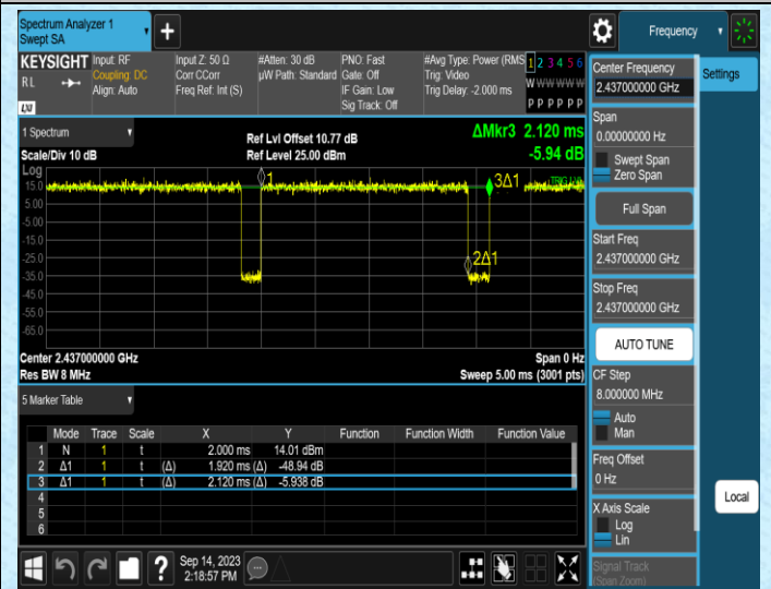
NTNV-11N20MIMO-Ant2-2437
