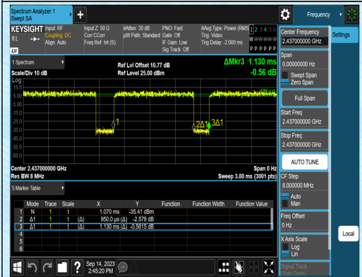
NTNV-11N40MIMO-Ant1-2437
