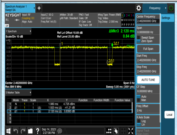
NTNV-11N20MIMO-Ant1-2462
