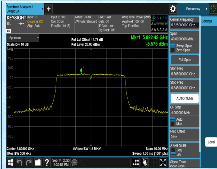
11N20MIMO-Ant1-5825
