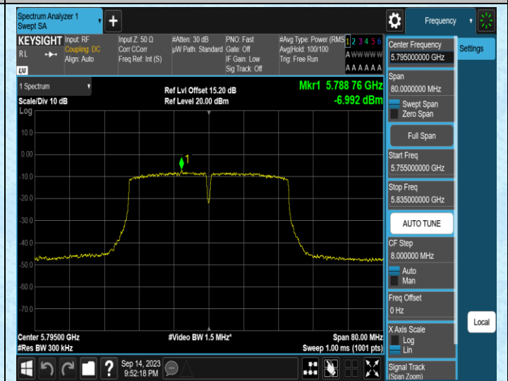
11N40MIMO-Ant2-5795
