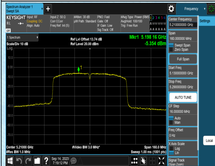
11AC80SISO-Ant1-5210
