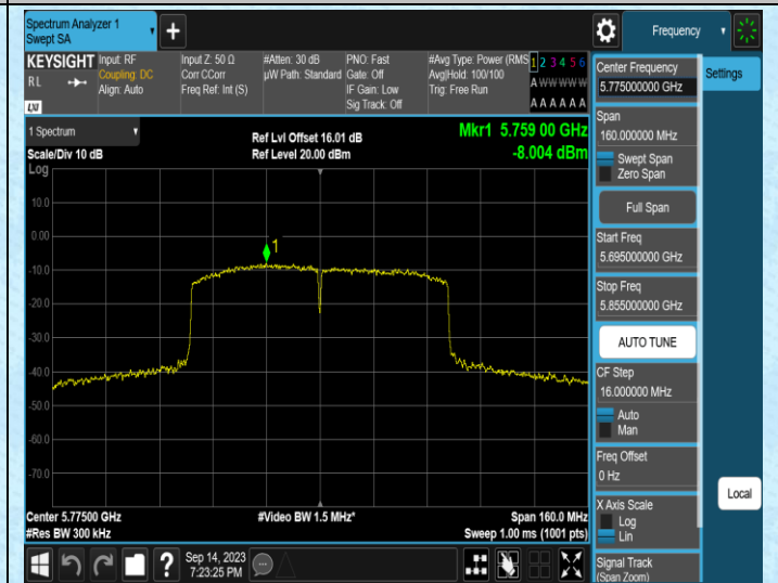
11AC80SISO-Ant1-5775
