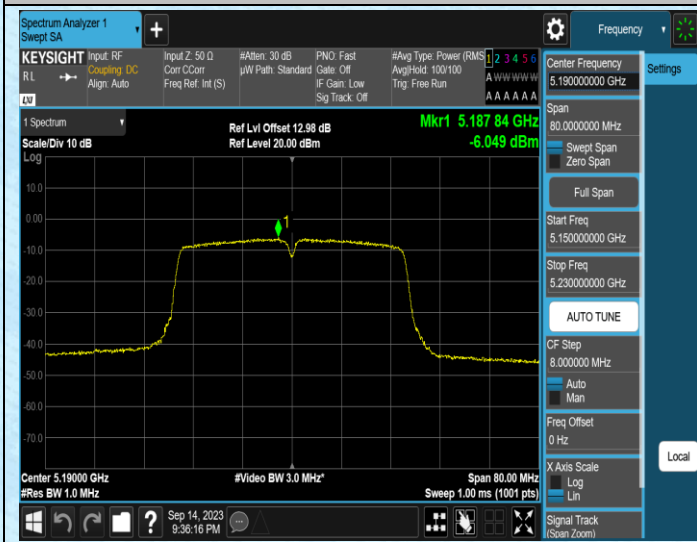
11N40MIMO-Ant1-5190
