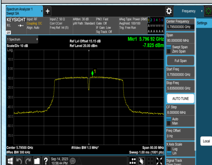
11AC40MIMO-Ant1-5795
