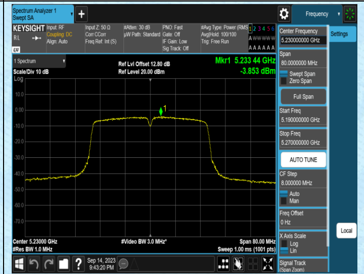
11N40MIMO-Ant2-5230
