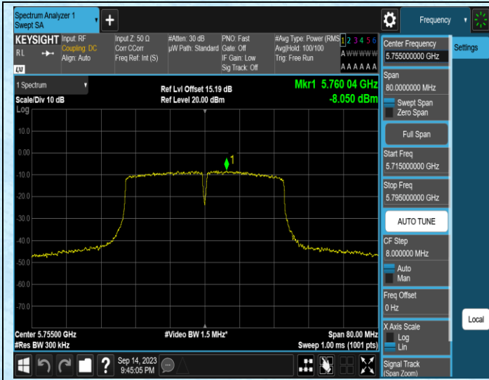
11N40MIMO-Ant1-5755
