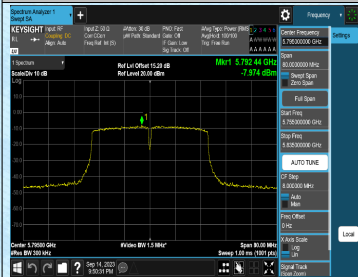
11N40MIMO-Ant1-5795
