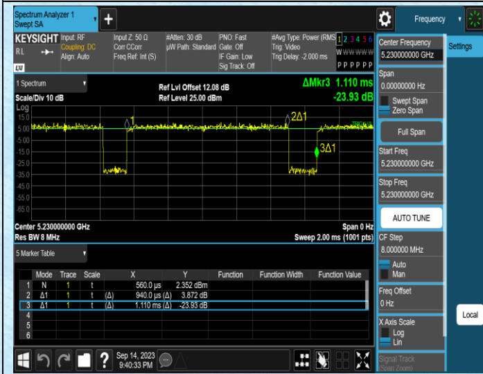
NTNV-11N40MIMO-Ant1-5230
