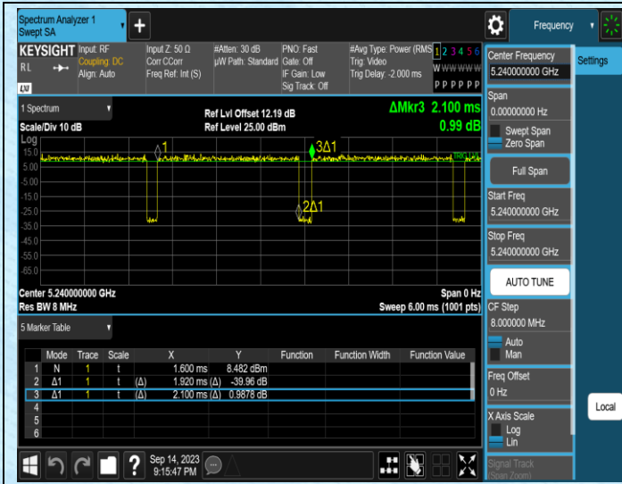
NTNV-11N20MIMO-Ant1-5240
