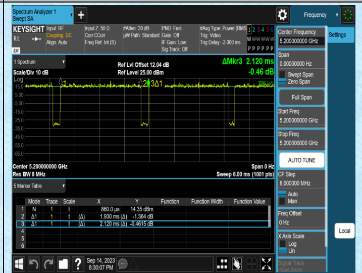
NTVN-11AC20SISO-Ant2-5200
