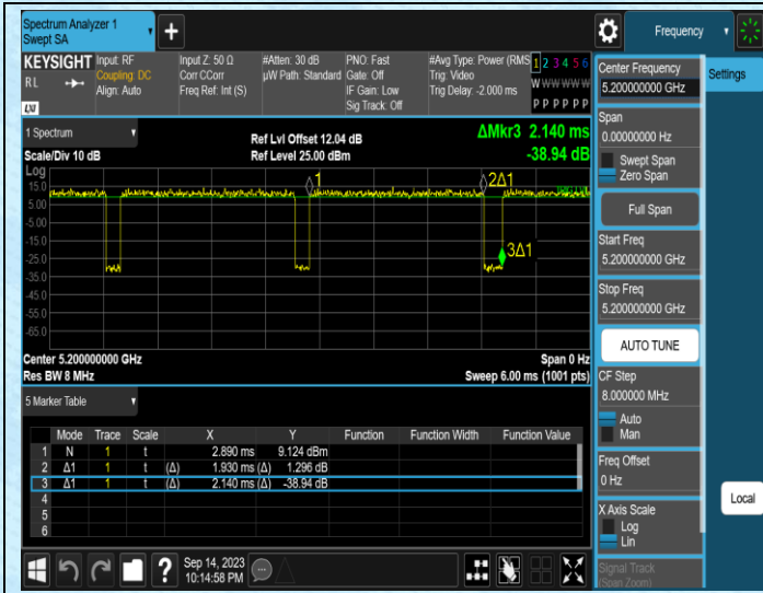
NTNV-11AC20MIMO-Ant1-5200
