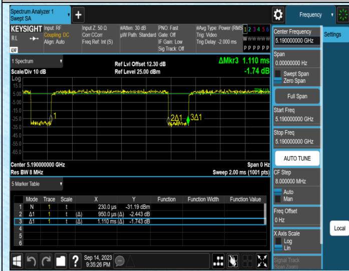
NTNV-11N40MIMO-Ant1-5190
