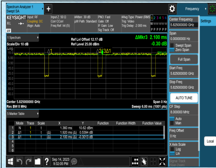
NTNV-11N20MIMO-Ant1-5825
