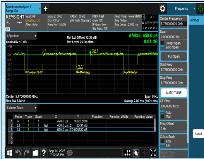
NTNV-11AC80SISO-Ant1-5775
