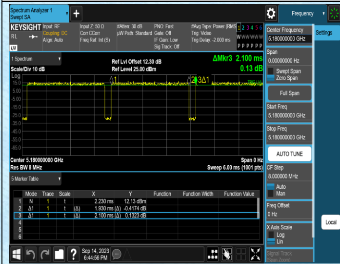
NTVN-11AC20SISO-Ant1-5180
