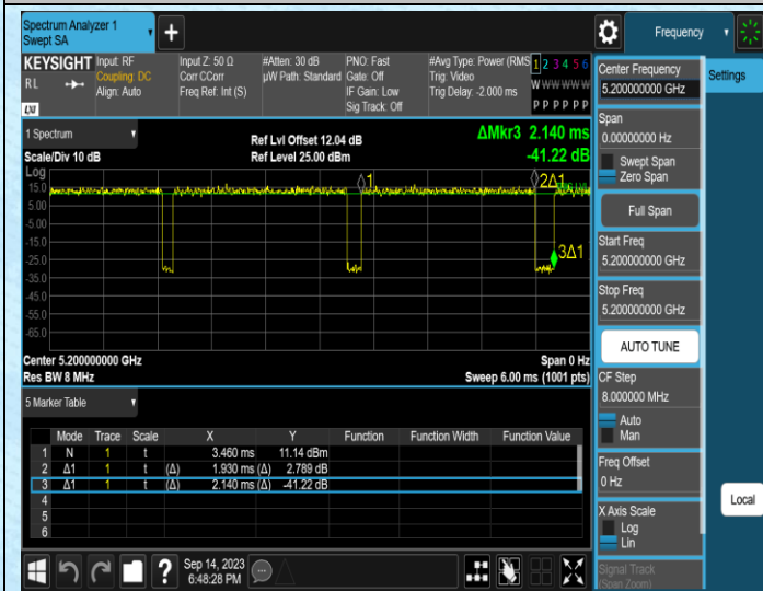
NTVN-11AC20SISO-Ant1-5200
