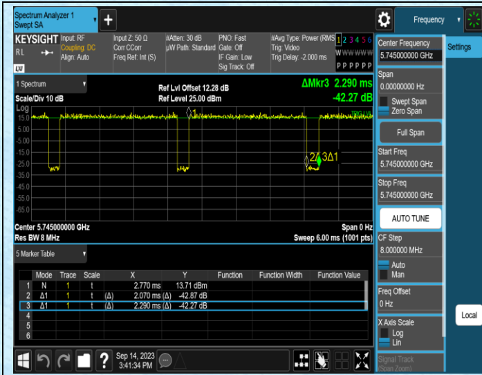
NTNV-11A-Ant1-5745
