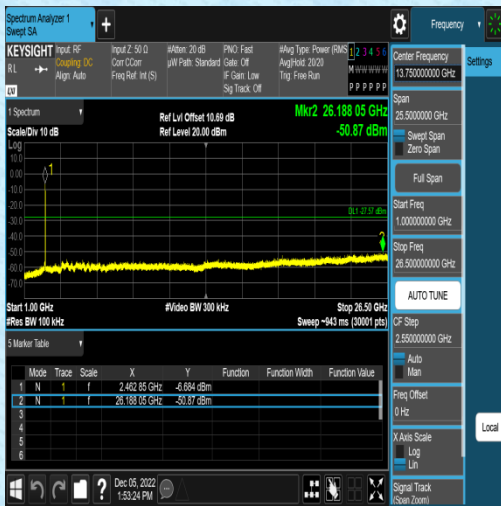
11N40SISO-Ant2-2422-30~1000~-6.17
