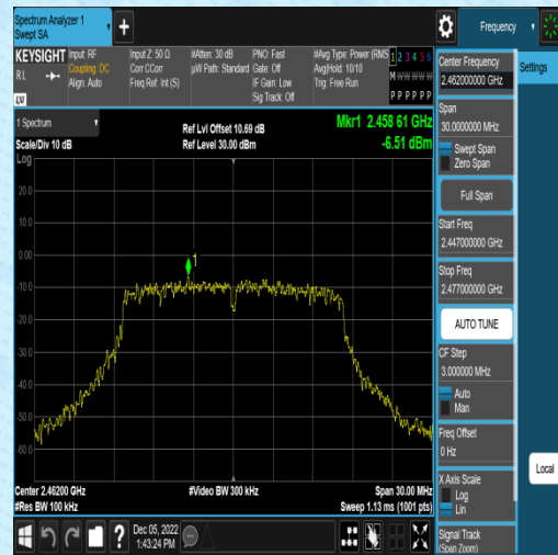
11G-Ant2-2462-1000~26500~-6.51
