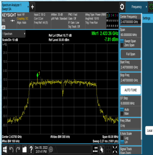
11N40SISO-Ant2-2437-1000~26500~-7.81
