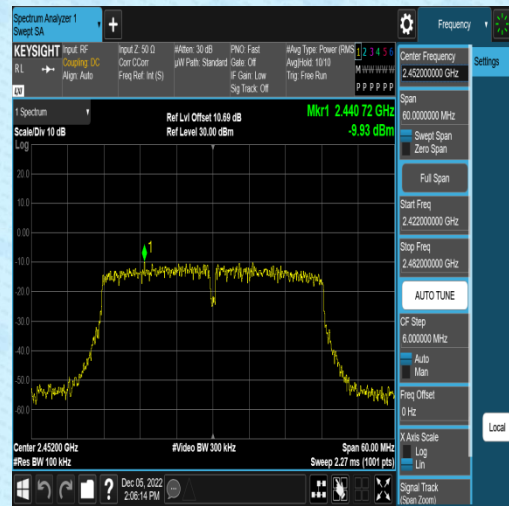
11N40SISO-Ant2-2452-1000~26500~-9.93
