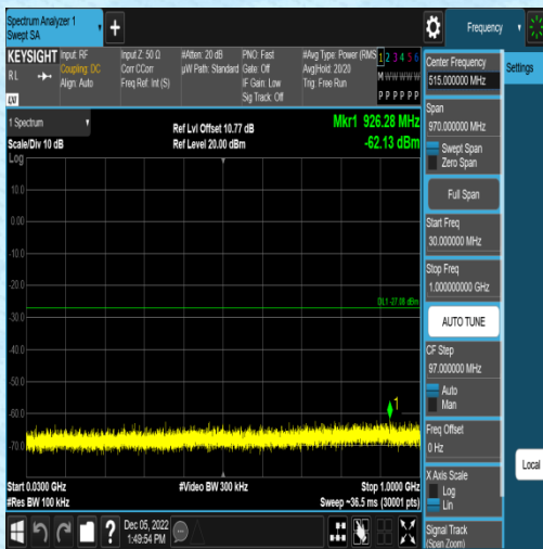
11N20SISO-Ant2-2462-0~Reference--7.57
