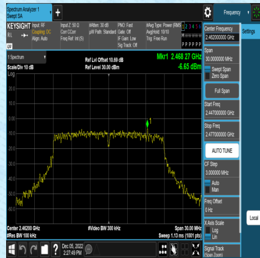
11N20MIMO-Ant2-2462-1000~26500~-6.65
