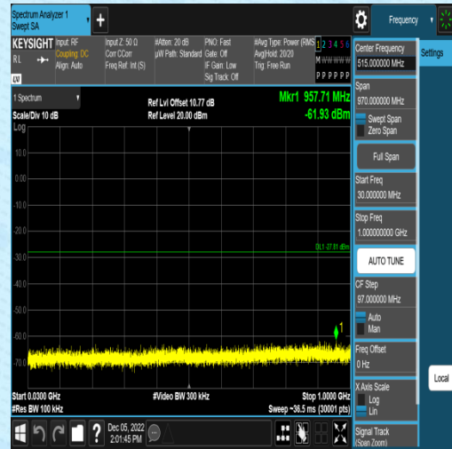
11N40SISO-Ant2-2452-0~Reference--9.93
