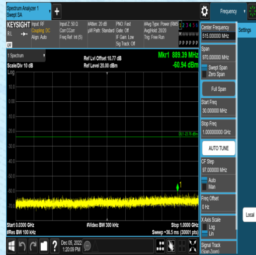
11N40SISO-Ant1-2452-0~Reference--8.13
