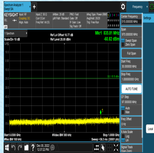
11G-Ant1-2462-0~Reference--1.49
