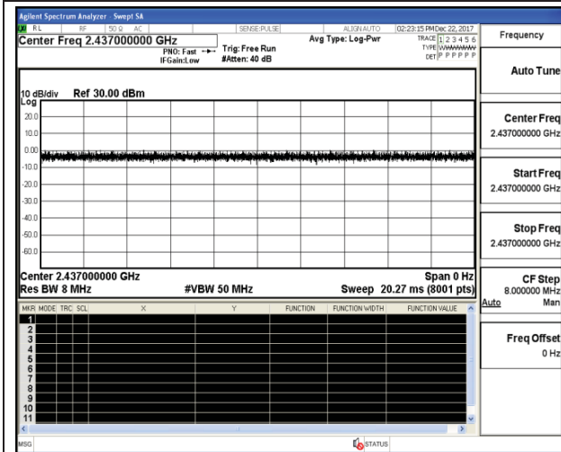
IEEE 802.11n HT20
