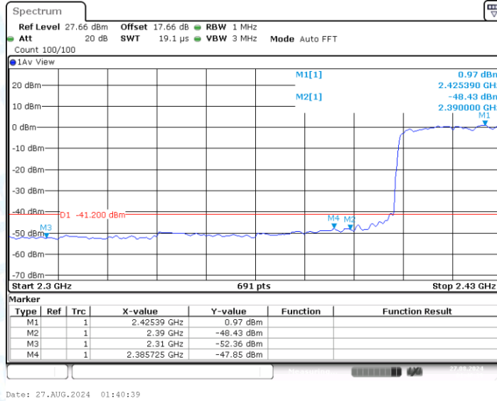
11AX40MIMO_Ant0_Low_2422_Peak
