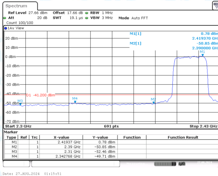
11AX20MIMO_Ant0_Low_2412_Peak
