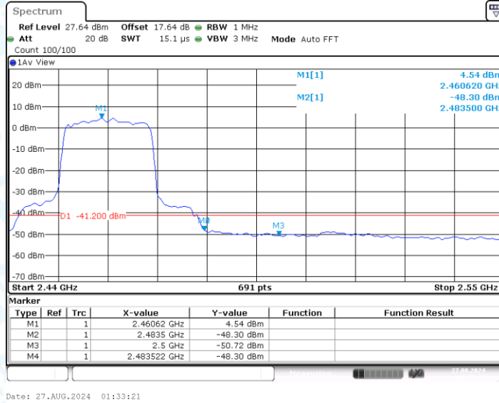
11AX20MIMO_Ant0_High_2462_Peak
