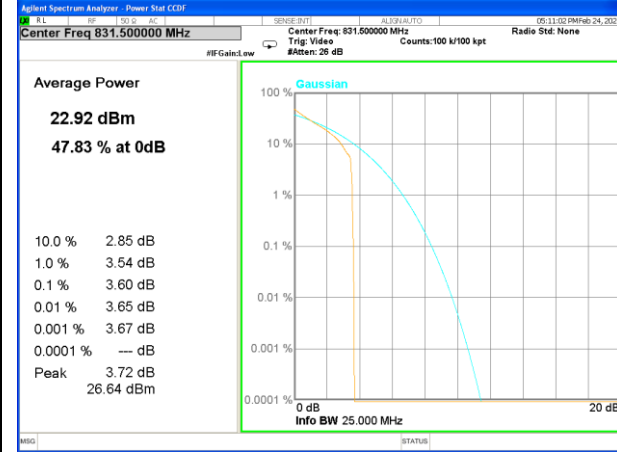
Band 26_1_Q16_Low
