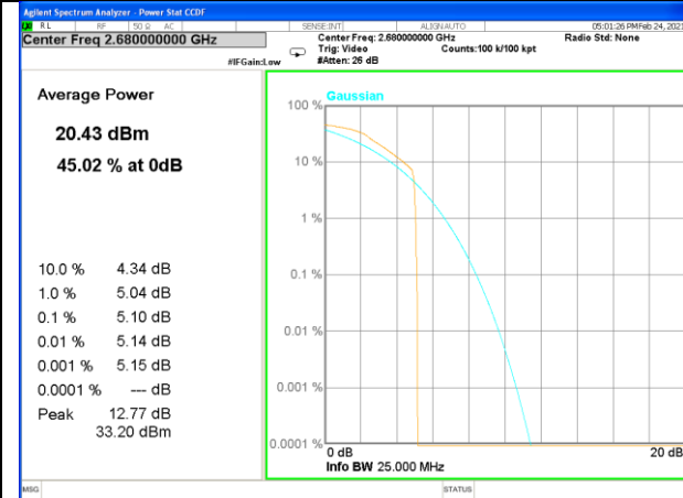
Band 41_1_Q16_High
