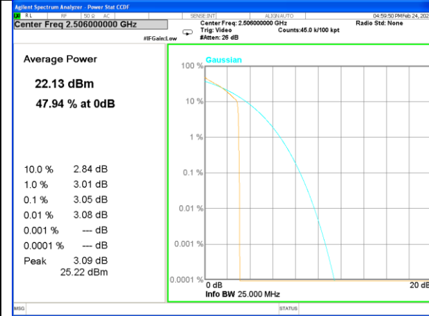
Band 41_1_Q16_Low
