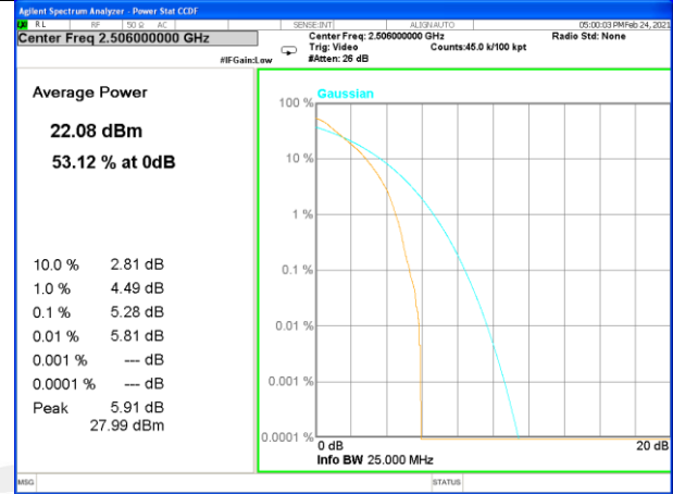
Band 41_100_Q16_Low
