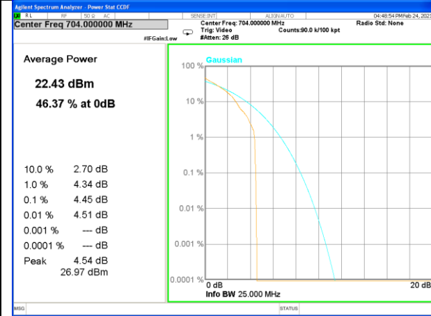
Band 12_1_Q16_Low
