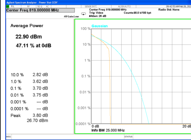
Band 26_1_Q16_Middle
