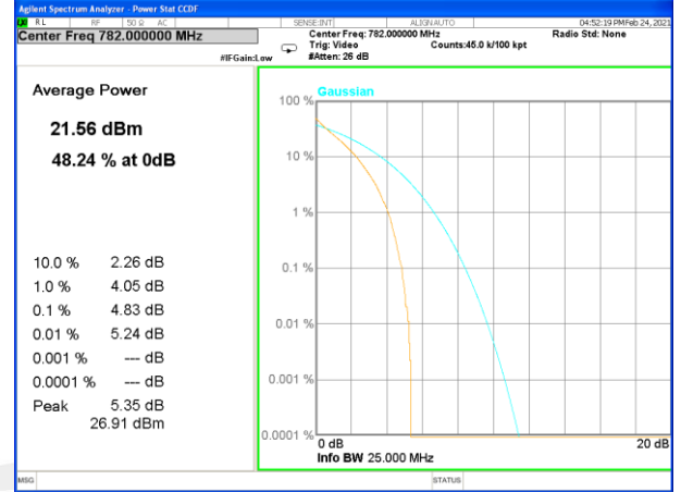
Band 13_50_Q16_Middle_
