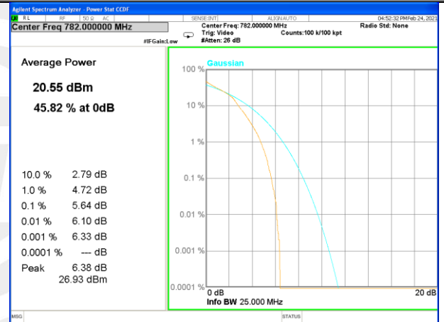
Band 13_50_Q16_Middle_
