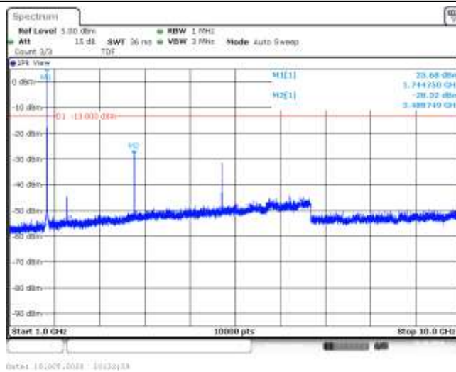
Band66-1.4MHz-QPSK-132322-1RB#0-Range2:1000~10000MHz--28.32-PASS
