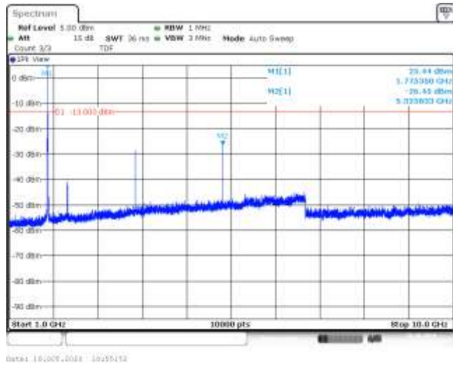
Band66-5MHz-QPSK-132647-1RB#0-Range2:1000~10000MHz--26.45-PASS
