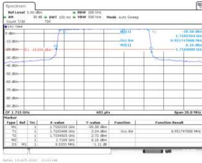
Band66-10MHz-QPSK-132022-50RB#0-8.952-9.533-PASS
