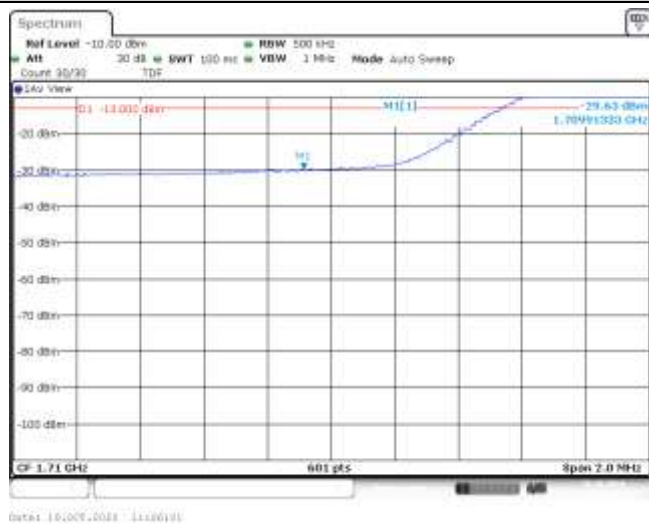
Band66-20MHz-QPSK-132072-100RB#0--29.63-PASS
