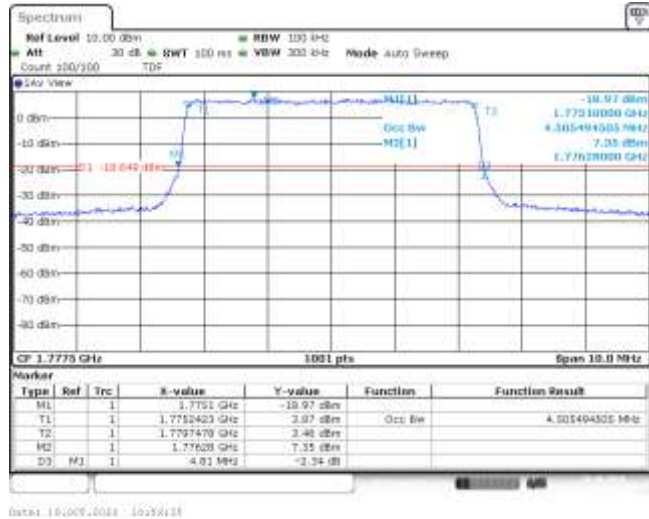
Band66-5MHz-QPSK-132647-25RB#0-4.505-4.810-PASS
