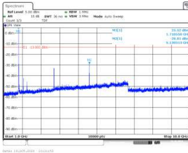
Band66-1.4MHz-QPSK-131979-1RB#0-Range2:1000~10000MHz--28.81-PASS
