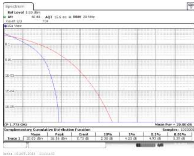
Band66-10MHz-QPSK-132622-50RB#0-4.93-13-PASS
