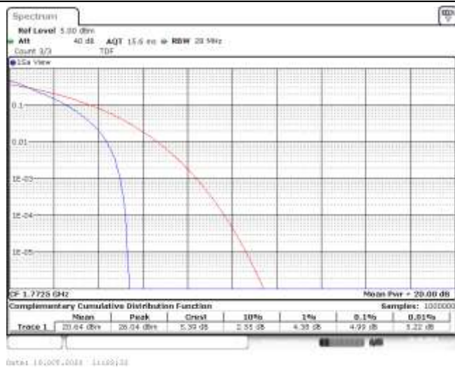
Band66-15MHz-QPSK-132597-75RB#0-4.99-13-PASS
