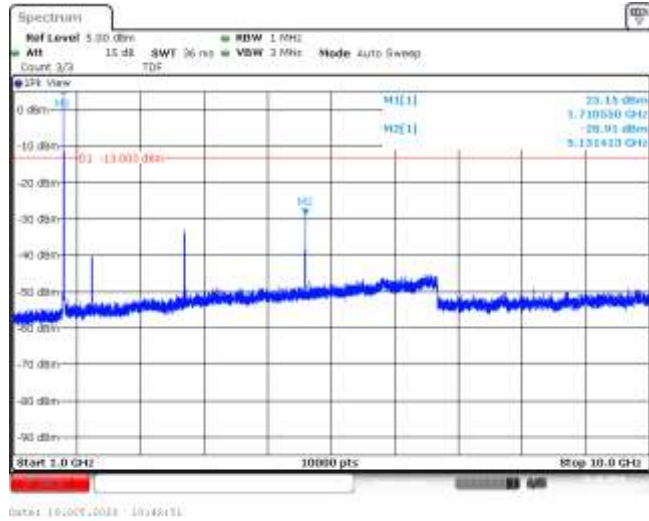
Band66-3MHz-16QAM-131987-1RB#0-Range2:1000~10000MHz--28.91-PASS
