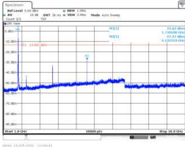
Band66-10MHz-QPSK-132022-1RB#0-Range2:1000~10000MHz--27.57-PASS
