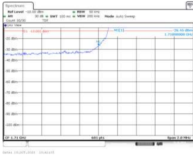
Band66-3MHz-QPSK-131987-15RB#0--26.45-PASS
