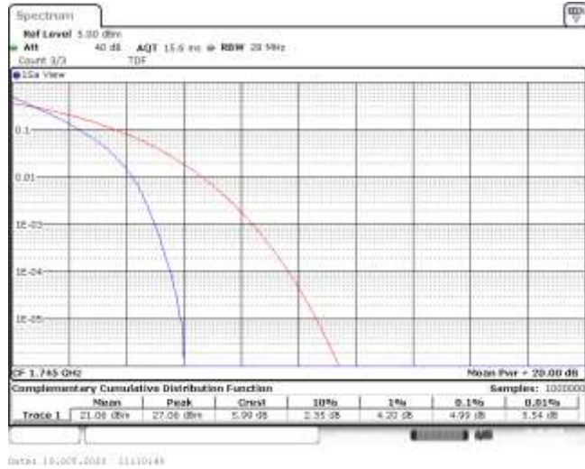
Band66-10MHz-QPSK-132322-50RB#0-4.99-13-PASS
