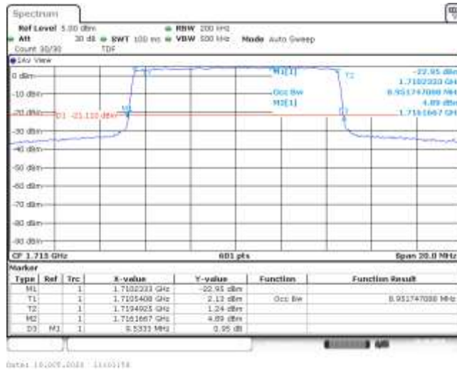
Band66-10MHz-16QAM-132022-50RB#0-8.952-9.533-PASS
