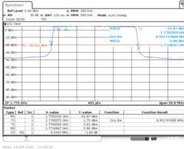
Band66-10MHz-QPSK-132622-50RB#0-8.952-9.533-PASS
