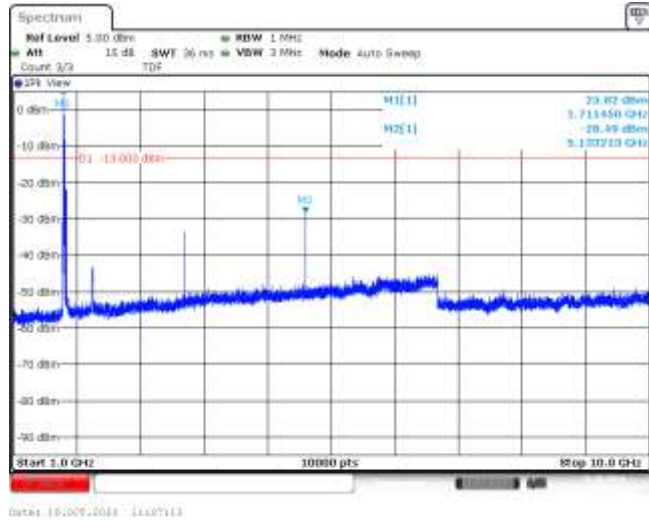
Band66-20MHz-QPSK-132072-1RB#0-Range2:1000~10000MHz--28.49-PASS
