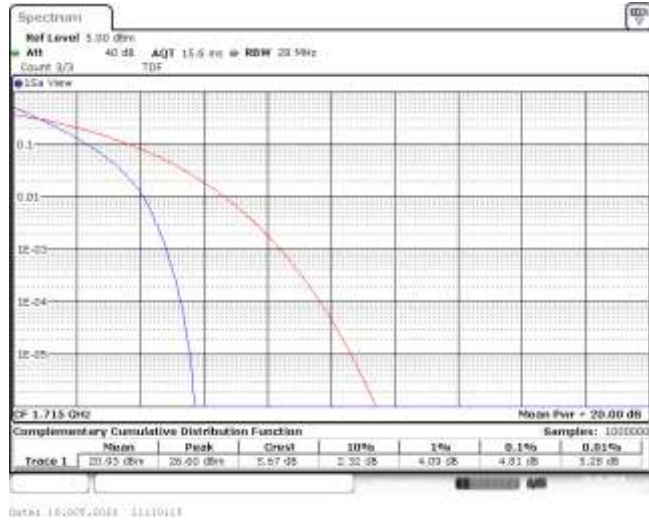
Band66-10MHz-QPSK-132022-50RB#0-4.81-13-PASS
