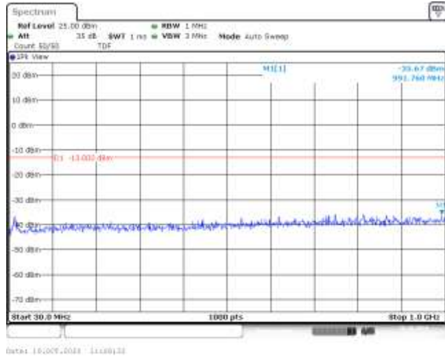
Band66-20MHz-QPSK-132572-1RB#0-Range1:30~1000MHz--35.67-PASS
