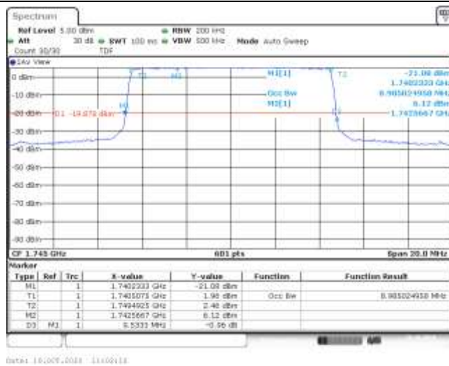
Band66-10MHz-QPSK-132322-50RB#0-8.985-9.533-PASS
