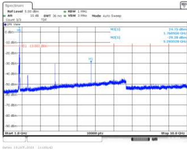
Band66-20MHz-QPSK-132572-1RB#0-Range2:1000~10000MHz--29.28-PASS
