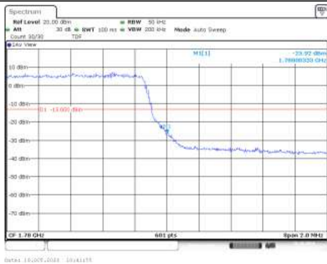
Band66-3MHz-QPSK-132657-15RB#0--25.92-PASS
