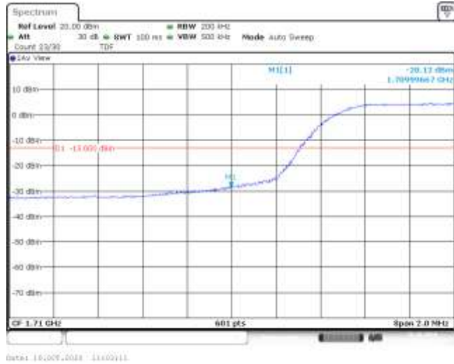
Band66-10MHz-QPSK-132022-50RB#0--28.12-PASS
