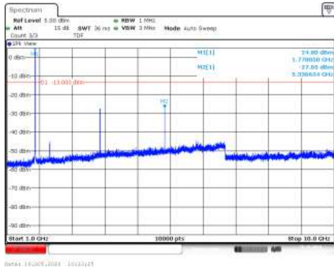
Band66-1.4MHz-QPSK-132665-1RB#0-Range2:1000~10000MHz--27.05-PASS
