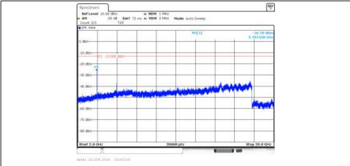
Band25-10MHz-QPSK-26365-1RB#0-Range1:30~1000MHz
