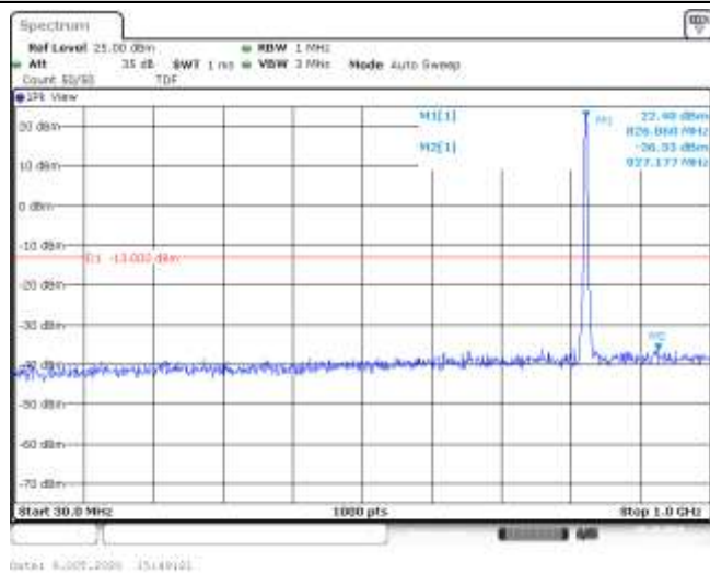
Band5-3MHz-QPSK-20415-15RB#0-Range1:30~1000MHz--36.33-PASS
