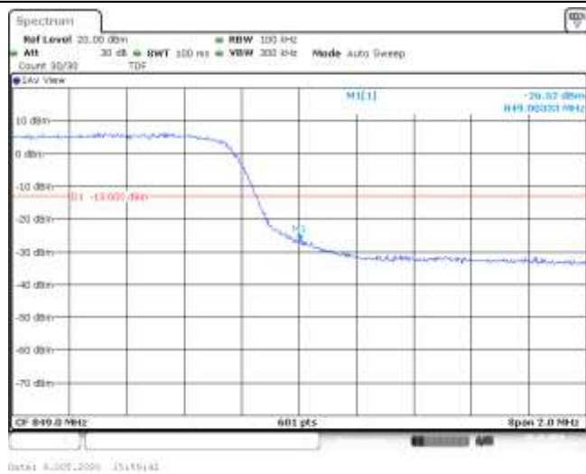
Band5-5MHz-QPSK-20625-25RB#0--26.52-PASS
