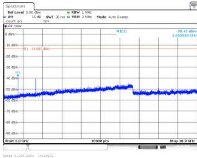
Band5-3MHz-QPSK-20415-15RB#0-Range2:1000~10000MHz--38.41-PASS
