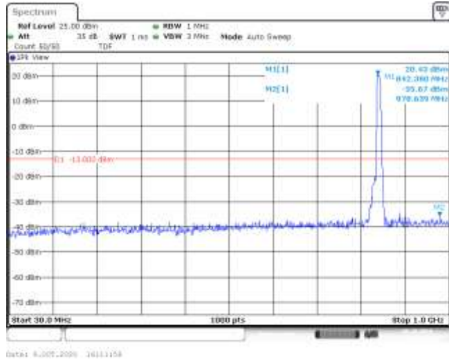
Band5-10MHz-QPSK-20600-50RB#0-Range1:30~1000MHz--35.67-PASS
