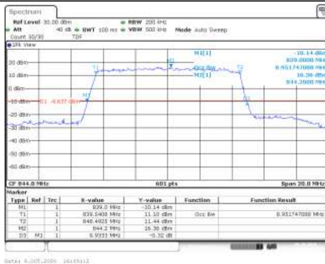
Band5-10MHz-QPSK-20600-50RB#0-8.952-9.933-PASS
