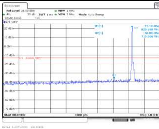
Band5-5MHz-QPSK-20425-25RB#0-Range1:30~1000MHz--36.09-PASS
