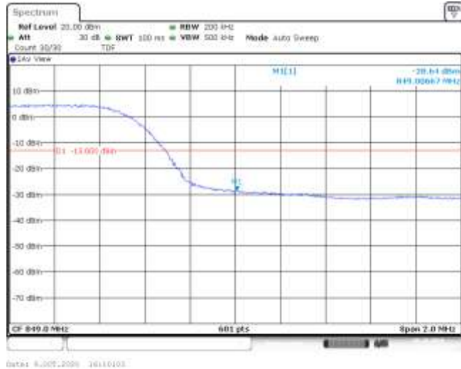
Band5-10MHz-QPSK-20600-50RB#0--28.64-PASS
