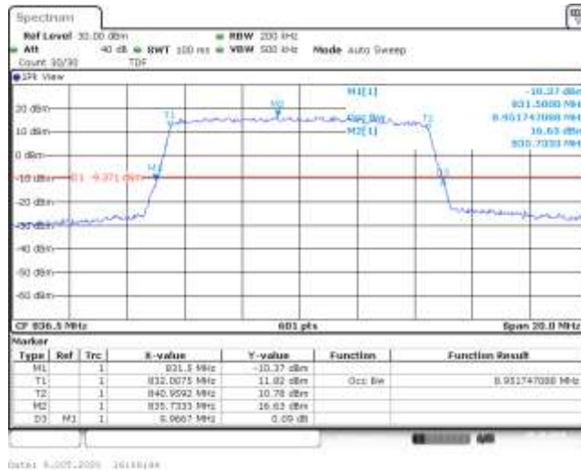
Band5-10MHz-QPSK-20525-50RB#0-8.952-9.967-PASS
