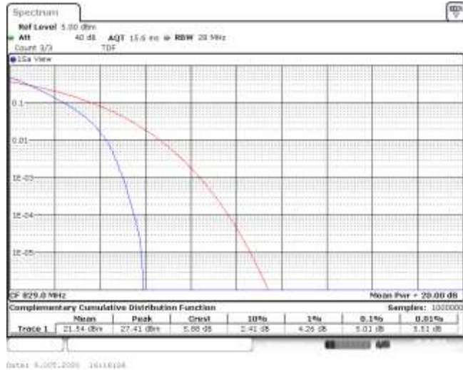
Band5-10MHz-QPSK-20450-50RB#0-5.01-13-PASS
