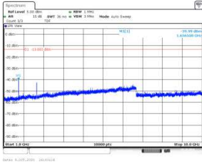
Band5-5MHz-QPSK-20425-25RB#0-Range2:1000~10000MHz--39.99-PASS
