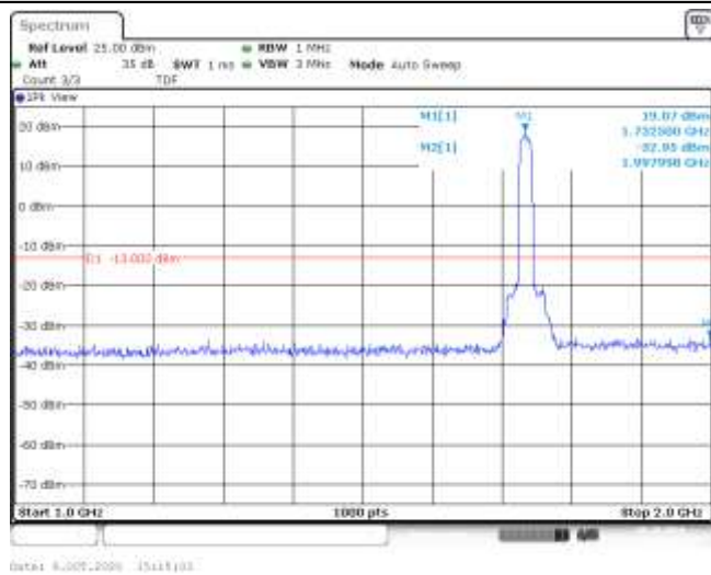
Band4-20MHz-QPSK-20175-100RB#0-Range2:1000~2000MHz--32.95-PASS
