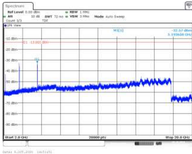
Band4-10MHz-QPSK-20175-50RB#0-Range3:2000~20000MHz--32.57-PASS
