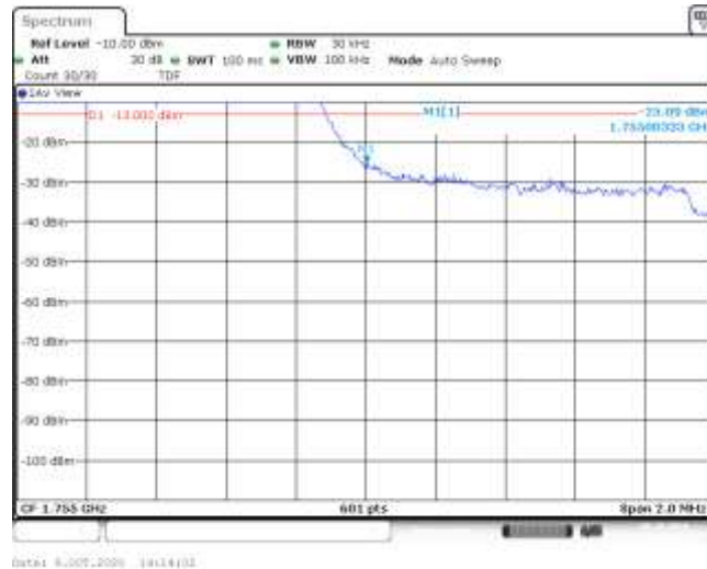
Band4-1.4MHz-QPSK-20393-6RB#0--25.09-PASS
