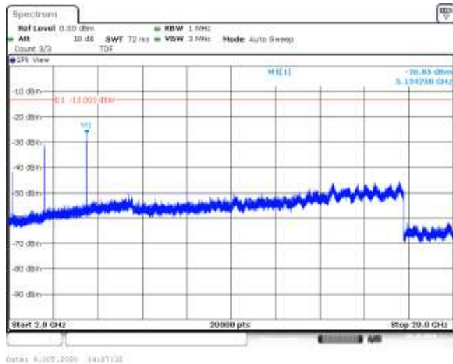
Band4-3MHz-QPSK-19965-15RB#0-Range3:2000~20000MHz--26.85-PASS
