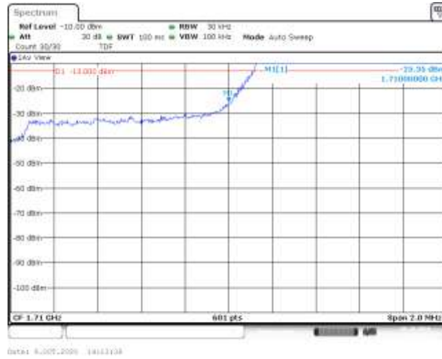
Band4-1.4MHz-QPSK-19957-6RB#0--25.35-PASS
