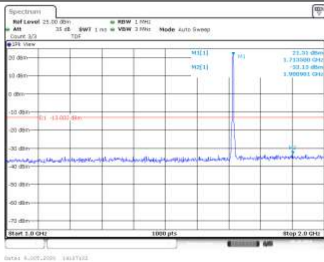
Band4-3MHz-QPSK-19965-15RB#0-Range2:1000~2000MHz--33.13-PASS
