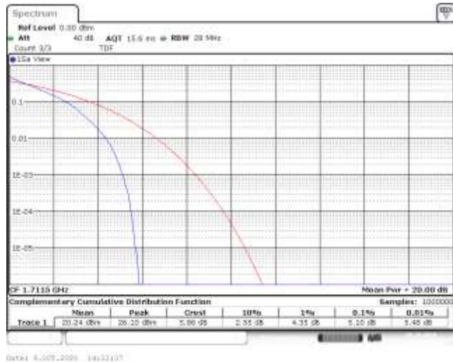
Band4-3MHz-QPSK-19965-15RB#0-5.10-13-PASS
