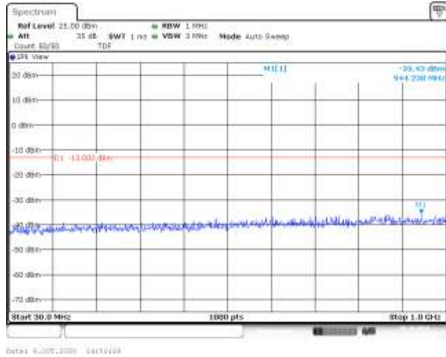
Band4-10MHz-QPSK-20000-50RB#0-Range1:30~1000MHz--35.43-PASS
