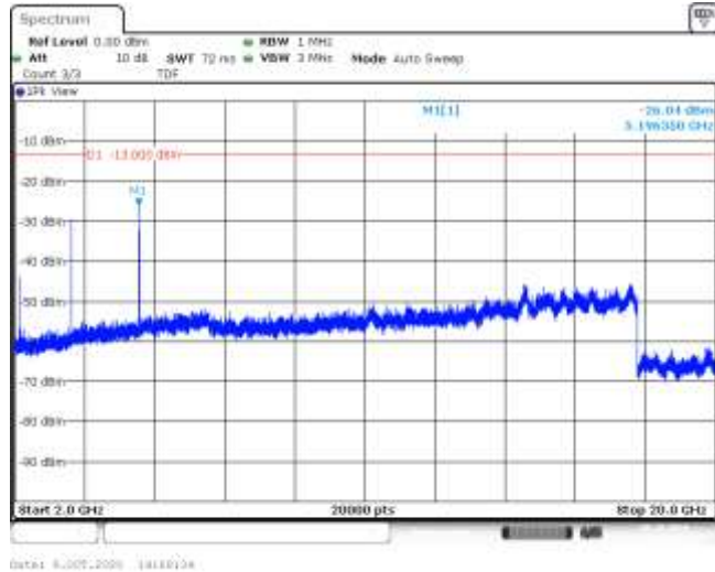
Band4-3MHz-QPSK-20175-15RB#0-Range3:2000~20000MHz--26.04-PASS
