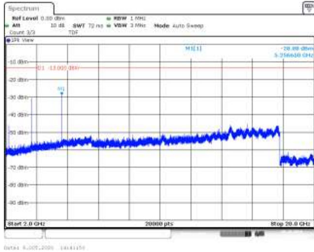
Band4-5MHz-QPSK-20375-25RB#0-Range3:2000~20000MHz--28.88-PASS
