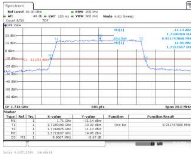
Band4-10MHz-QPSK-20000-50RB#0-8.952-9.967-PASS
