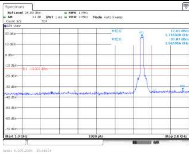
Band4-20MHz-QPSK-20300-100RB#0-Range2:1000~2000MHz--33.07-PASS
