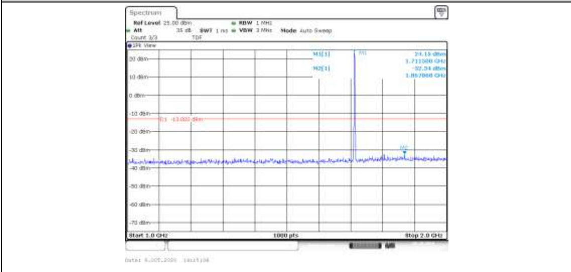
Band4-1.4MHz-16QAM-19957-6RB#0-Range2:1000~2000MHz--32.34-PASS
