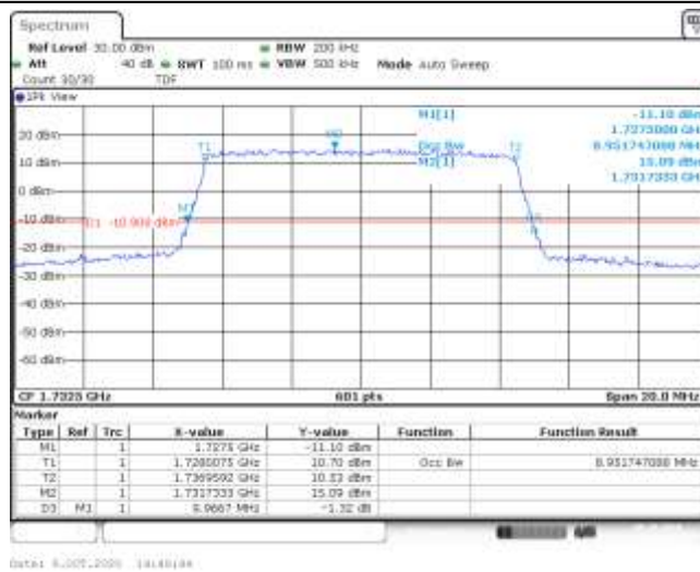
Band4-10MHz-QPSK-20175-50RB#0-8.952-9.967-PASS
