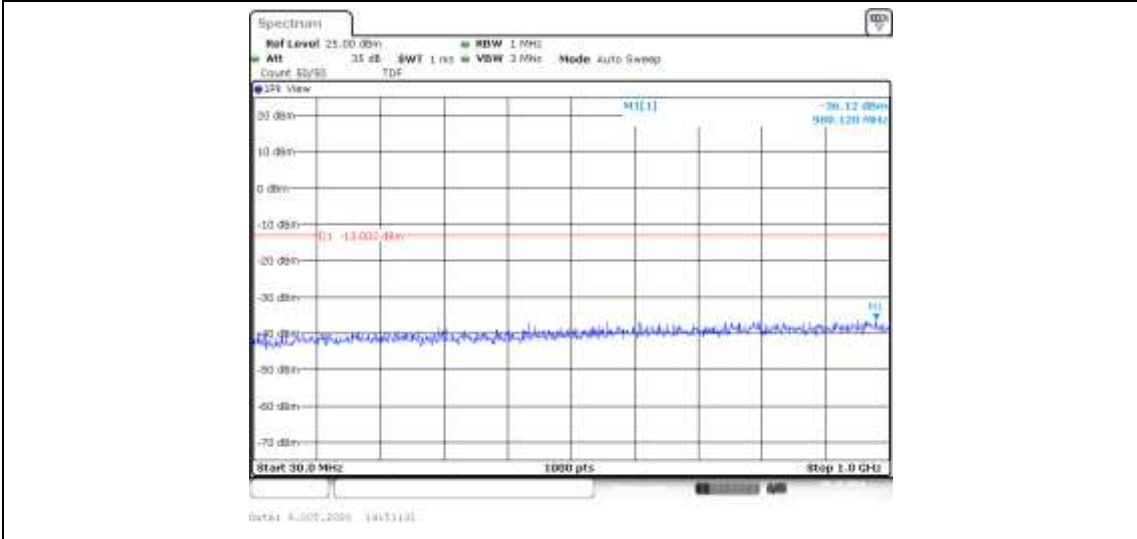
Band4-10MHz-QPSK-20175-50RB#0-Range1:30~1000MHz--36.12-PASS
