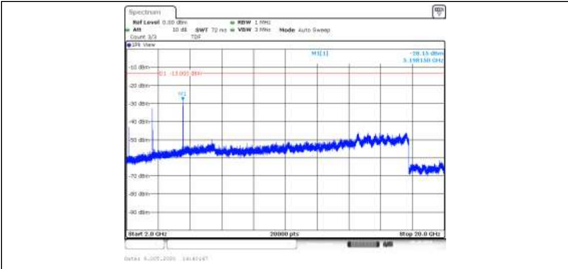
Band4-5MHz-QPSK-20175-25RB#0-Range3:2000~20000MHz--28.15-PASS
