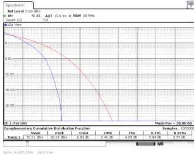
Band4-10MHz-QPSK-20000-50RB#0-5.04-13-PASS
