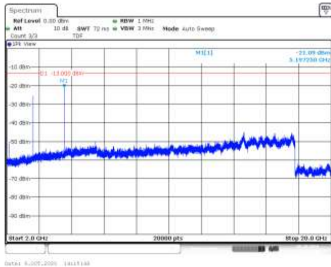
Band4-1.4MHz-QPSK-20175-6RB#0-Range3:2000~20000MHz--21.09-PASS
