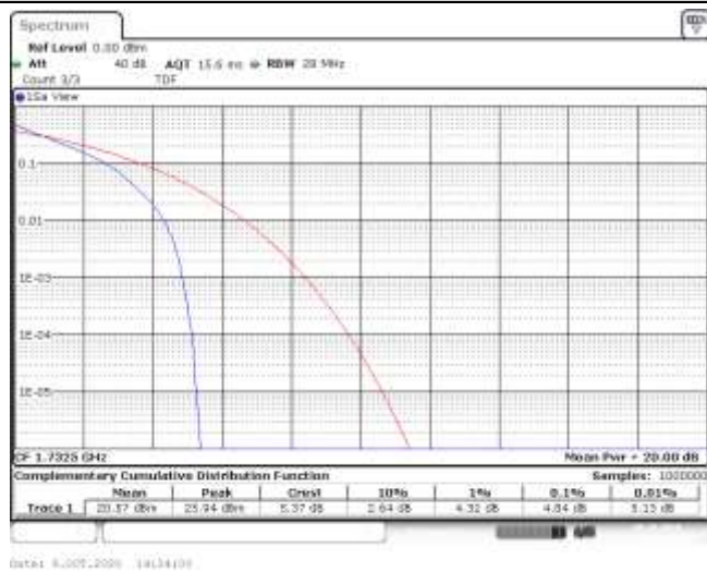
Band4-3MHz-QPSK-20175-15RB#0-4.84-13-PASS
