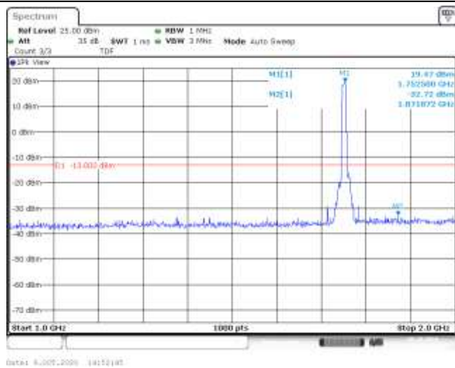
Band4-10MHz-QPSK-20350-50RB#0-Range2:1000~2000MHz--32.72-PASS
