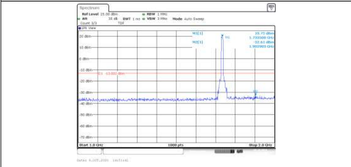
Band4-10MHz-QPSK-20175-50RB#0-Range2:1000~2000MHz--32.61-PASS
