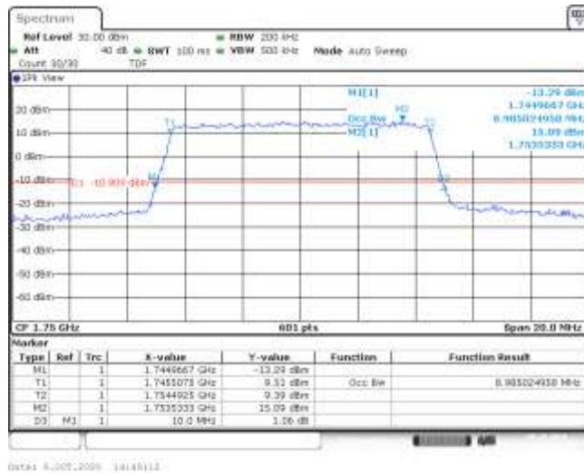
Band4-10MHz-QPSK-20350-50RB#0-8.985-10.000-PASS
