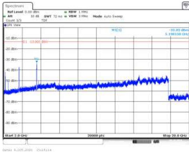
Band4-20MHz-QPSK-20175-100RB#0-Range3:2000~20000MHz--33.03-PASS
