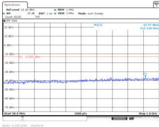
Band4-3MHz-QPSK-20385-15RB#0-Range1:30~1000MHz--35.97-PASS
