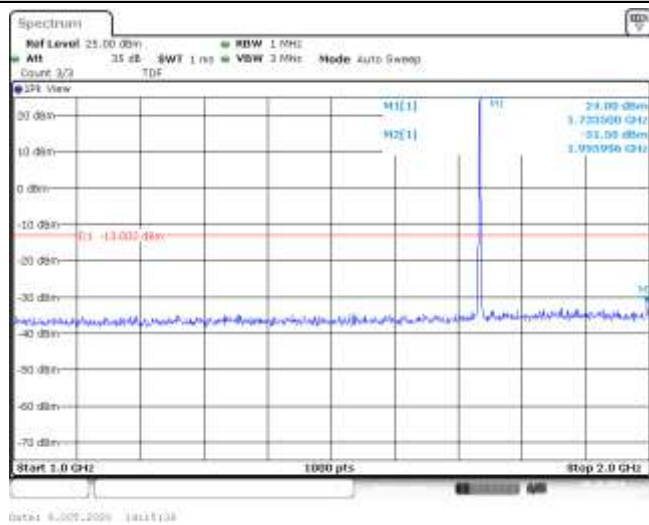
Band4-1.4MHz-QPSK-20175-6RB#0-Range2:1000~2000MHz--31.5-PASS
