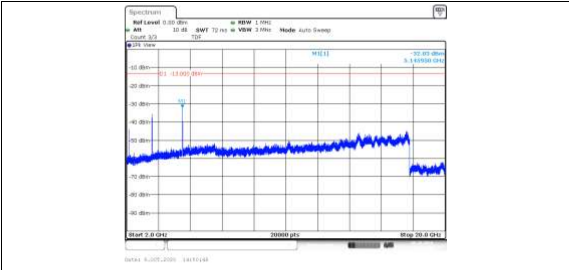
Band4-10MHz-QPSK-20000-50RB#0-Range3:2000~20000MHz--32.03-PASS
