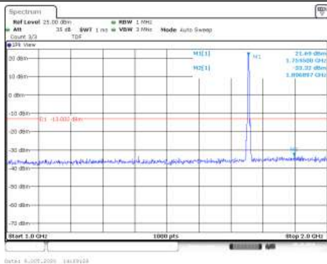
Band4-3MHz-QPSK-20385-15RB#0-Range2:1000~2000MHz--33.32-PASS
