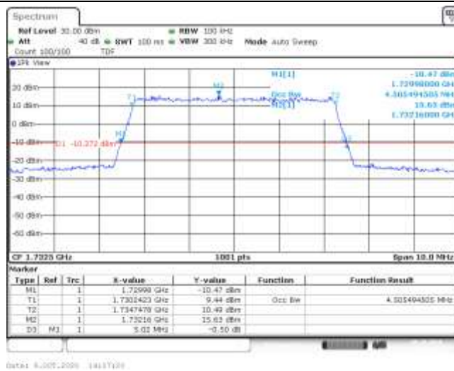
Band4-5MHz-QPSK-20175-25RB#0-4.505-5.020-PASS
