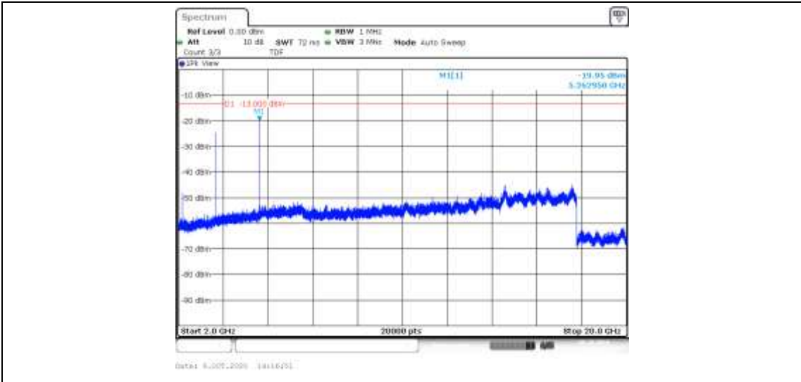
Band4-1.4MHz-QPSK-20393-6RB#0-Range3:2000~20000MHz--19.95-PASS
