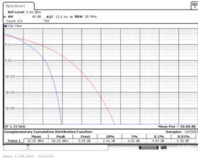
Band4-20MHz-QPSK-20050-100RB#0-4.93-13-PASS
