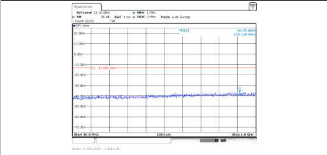
Band4-5MHz-QPSK-20375-25RB#0-Range1:30~1000MHz--36.35-PASS
