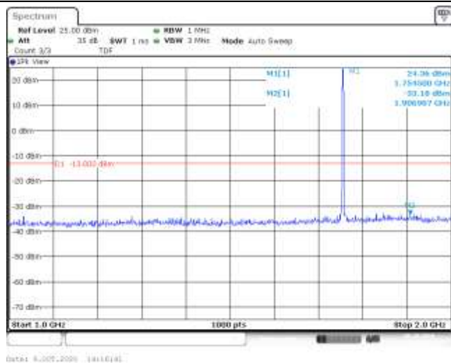
Band4-1.4MHz-QPSK-20393-6RB#0-Range2:1000~2000MHz--33.18-PASS
