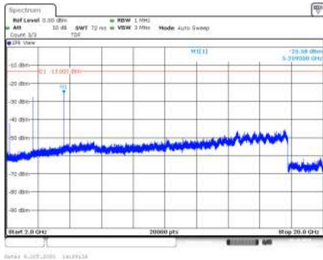
Band4-3MHz-QPSK-20385-15RB#0-Range3:2000~20000MHz--25.58-PASS
