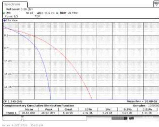
Band4-20MHz-QPSK-20300-100RB#0-5.04-13-PASS
