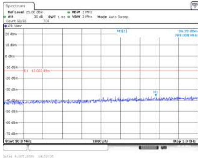
Band4-10MHz-QPSK-20350-50RB#0-Range1:30~1000MHz--36.2-PASS
