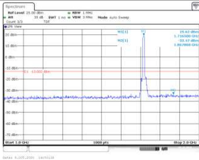
Band4-10MHz-QPSK-20000-50RB#0-Range2:1000~2000MHz--33.47-PASS
