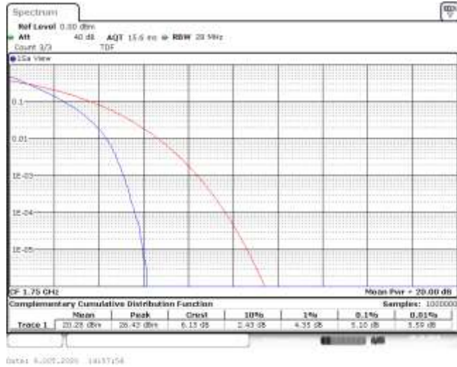
Band4-10MHz-QPSK-20350-50RB#0-5.10-13-PASS
