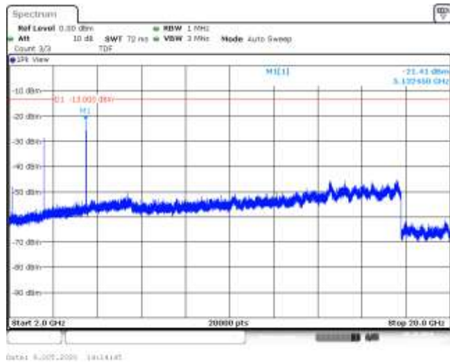
Band4-1.4MHz-QPSK-19957-6RB#0-Range3:2000~20000MHz--21.41-PASS
