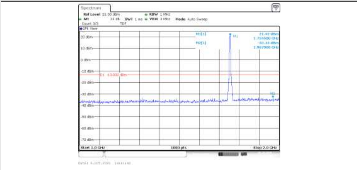
Band4-5MHz-QPSK-20375-25RB#0-Range2:1000~2000MHz--33.15-PASS
