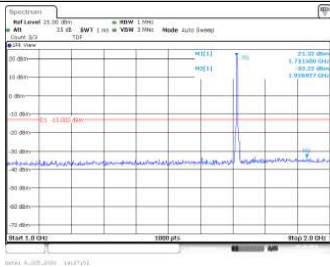
Band4-3MHz-16QAM-19965-15RB#0-Range2:1000~2000MHz--33.22-PASS
