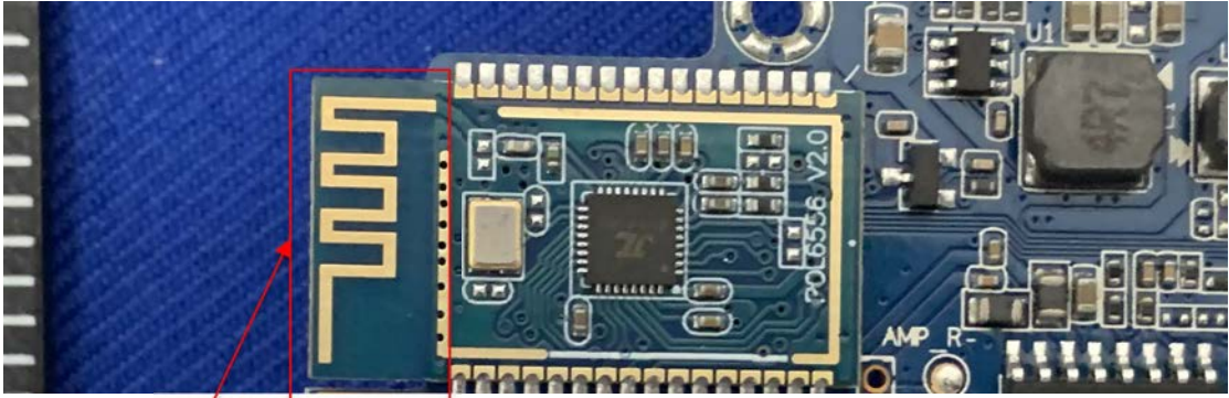
EUT Photo
