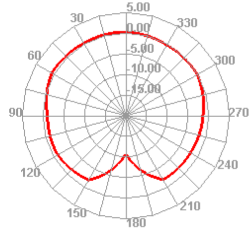
2410.000MHz E2
