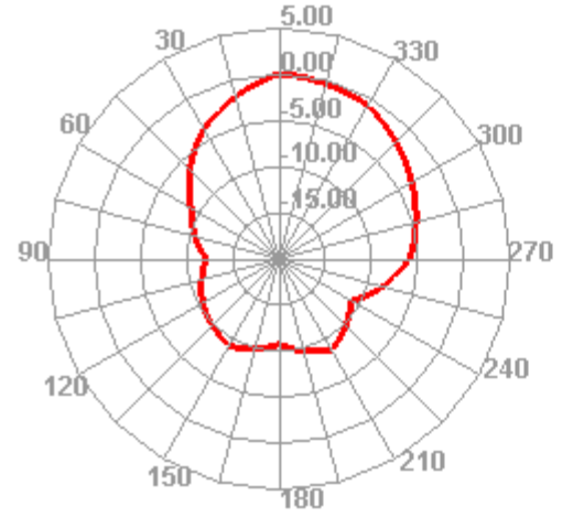
2410.000MHz E1
