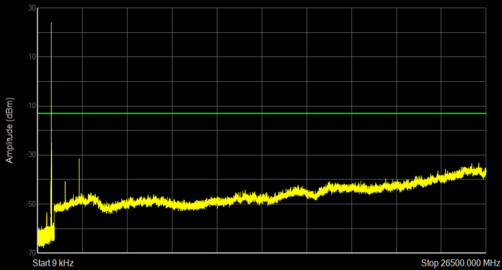
Band26(824-849) QPSK BW=15MHz Channel=26865 RB Size=1 Position=#0
