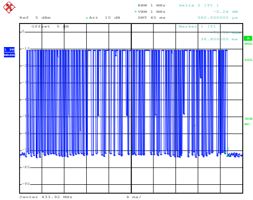
T 15=40ms:
