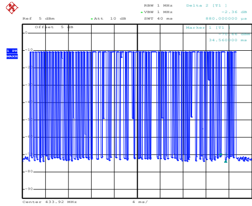
T 14=40ms:
