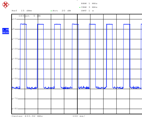
T period:
