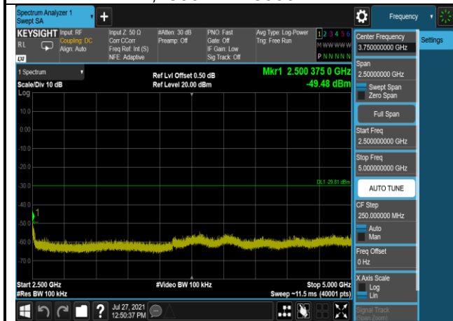
802.11n(HT40),2452MHz,Ant1,Plot 4,2500MHz~5000MHz
