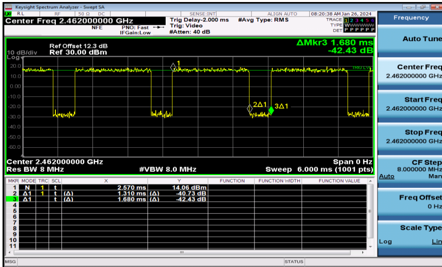
NTNV-11N20MIMO-Ant1-2462
