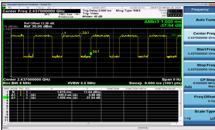
NTNV-11N40MIMO-Ant1-2437
