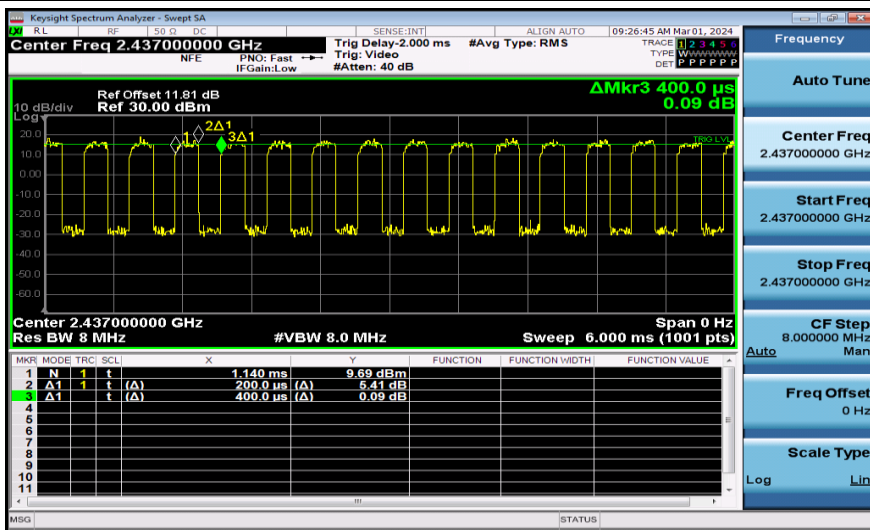
NTNV-11AX40MIMO-Ant1-2437
