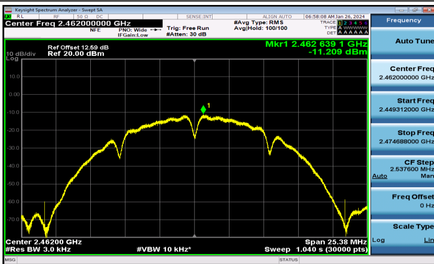
11B-Ant2-2462-PASS
