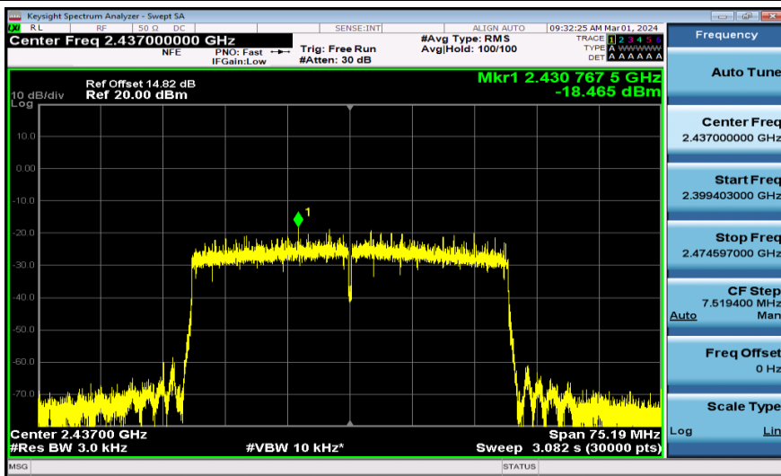
11AX40MIMO-Ant1-2437-PASS
