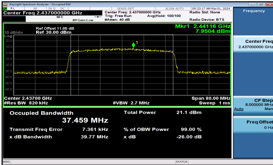
11AX40MIMO-Ant2-2437
