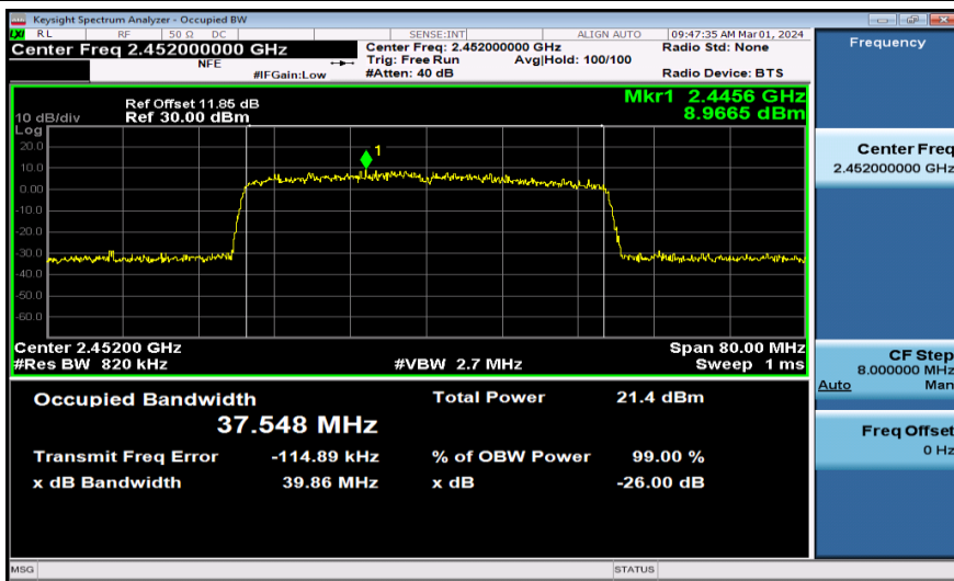
11AX40MIMO-Ant2-2452
