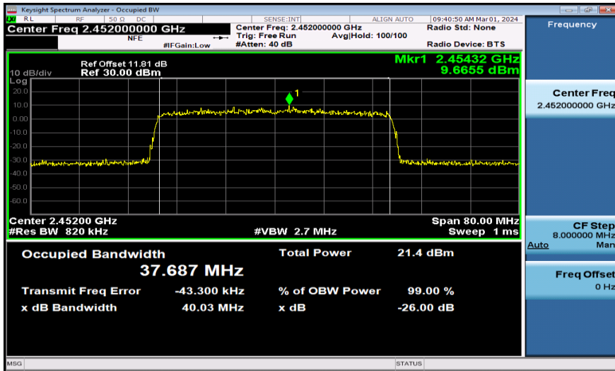
11AX40MIMO-Ant1-2452
