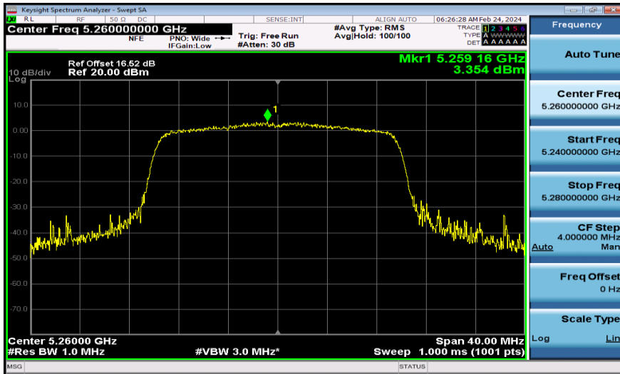
11AX20MIMO-Ant1-5260-PASS
