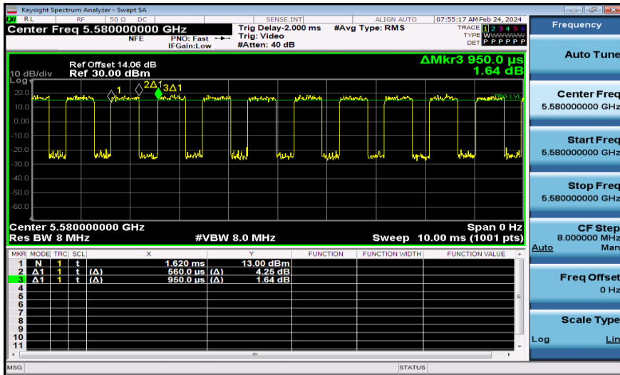
NTNV-11AX20MIMO-Ant1-5580
