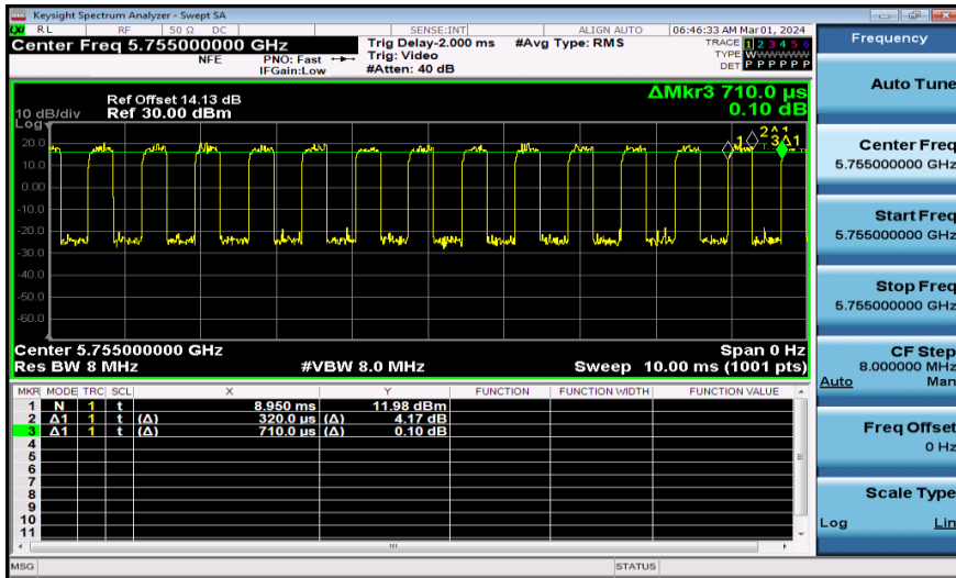
NTNV-11AX40MIMO-Ant1-5755
