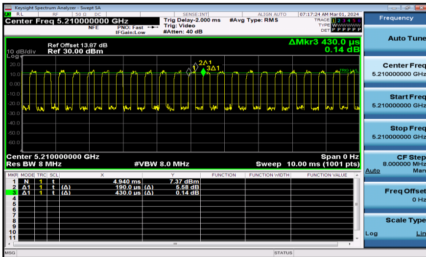
NTNV-11AX80MIMO-Ant1-5210
