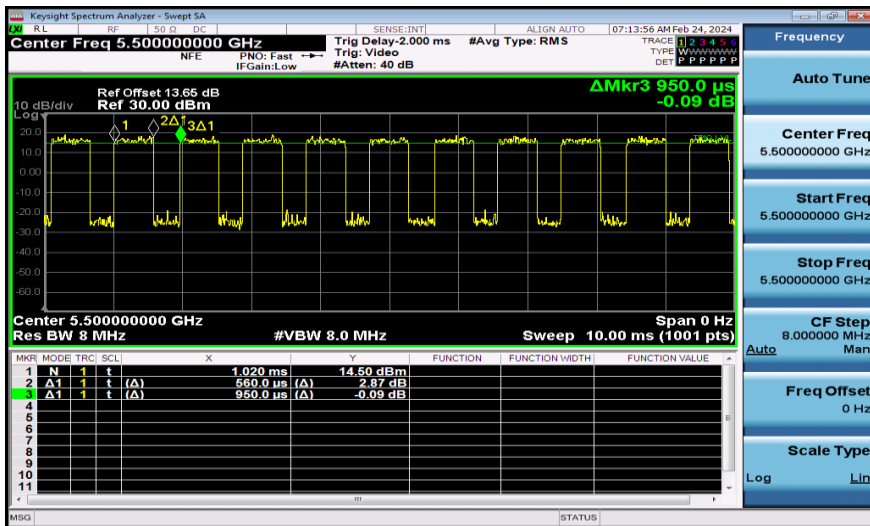
NTNV-11AX20MIMO-Ant1-5500
