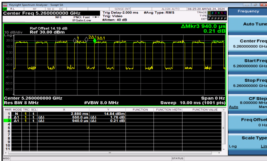
NTNV-11AX20MIMO-Ant1-5260
