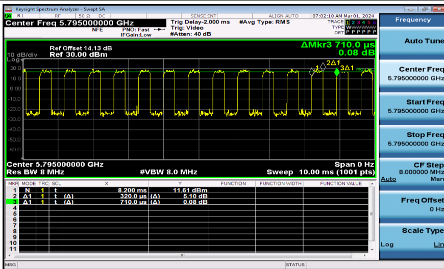
NTNV-11AX40MIMO-Ant1-5795
