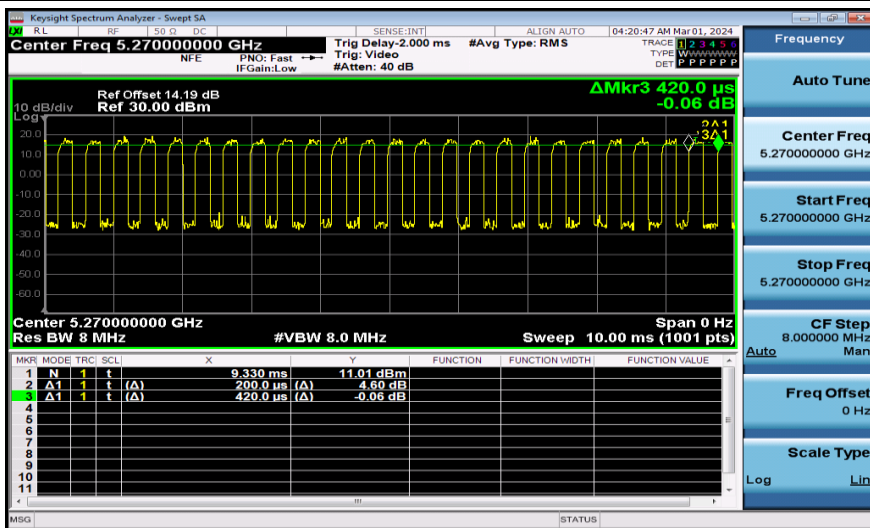
NTNV-11AX40MIMO-Ant1-5270
