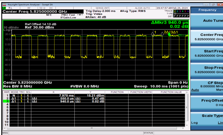
NTNV-11AX20MIMO-Ant1-5825
