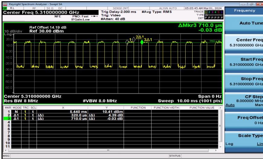
NTNV-11AX40MIMO-Ant1-5310
