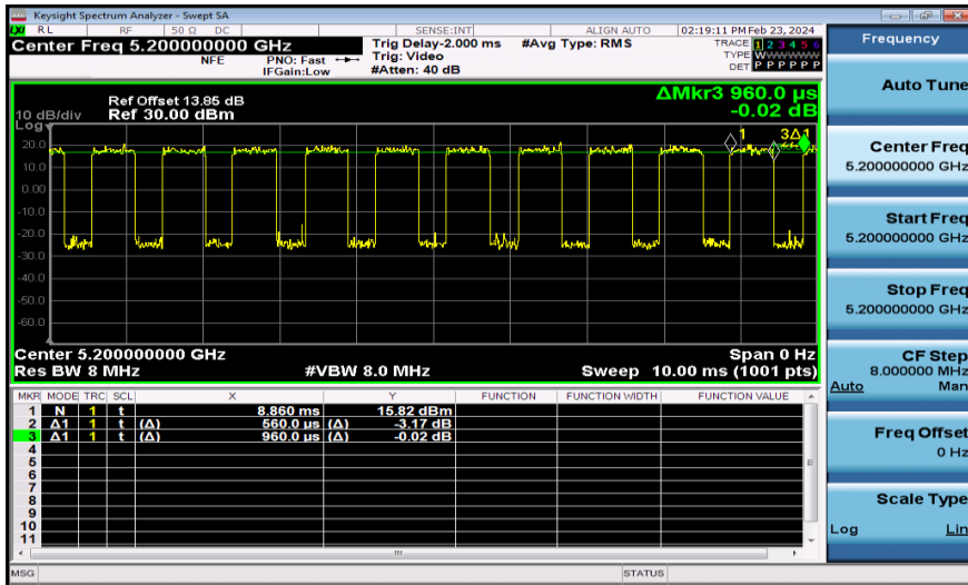
NTNV-11AX20MIMO-Ant2-5200
