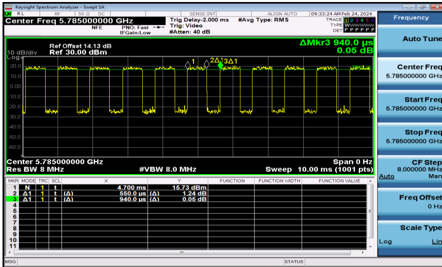
NTNV-11AX20MIMO-Ant1-5785
