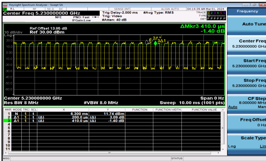
NTNV-11AX40MIMO-Ant2-5230
