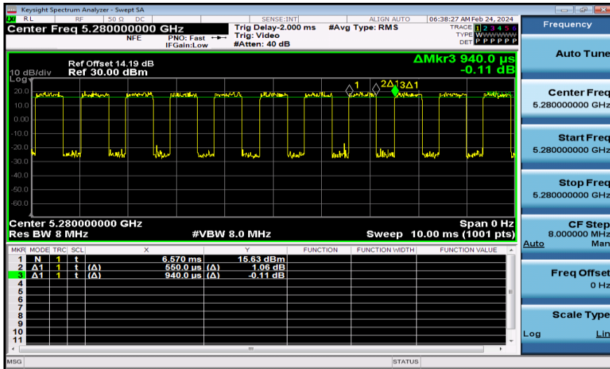
NTNV-11AX20MIMO-Ant1-5280
