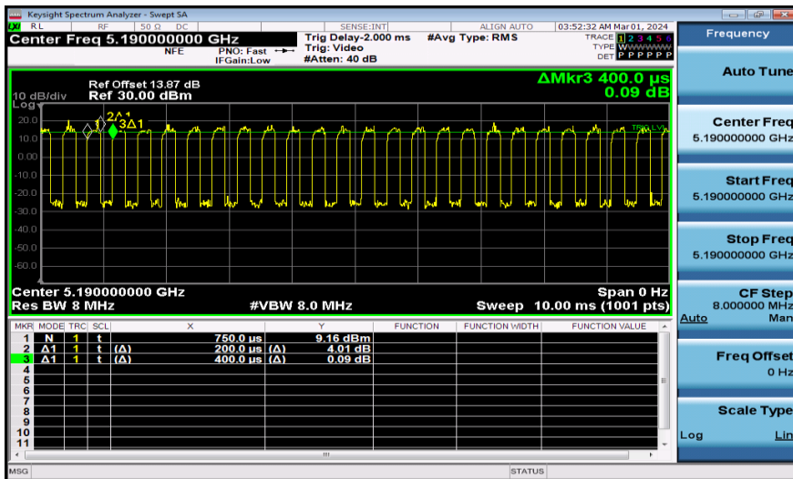
NTNV-11AX40MIMO-Ant1-5190
