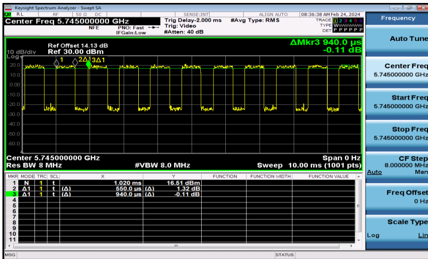
NTNV-11AX20MIMO-Ant1-5745
