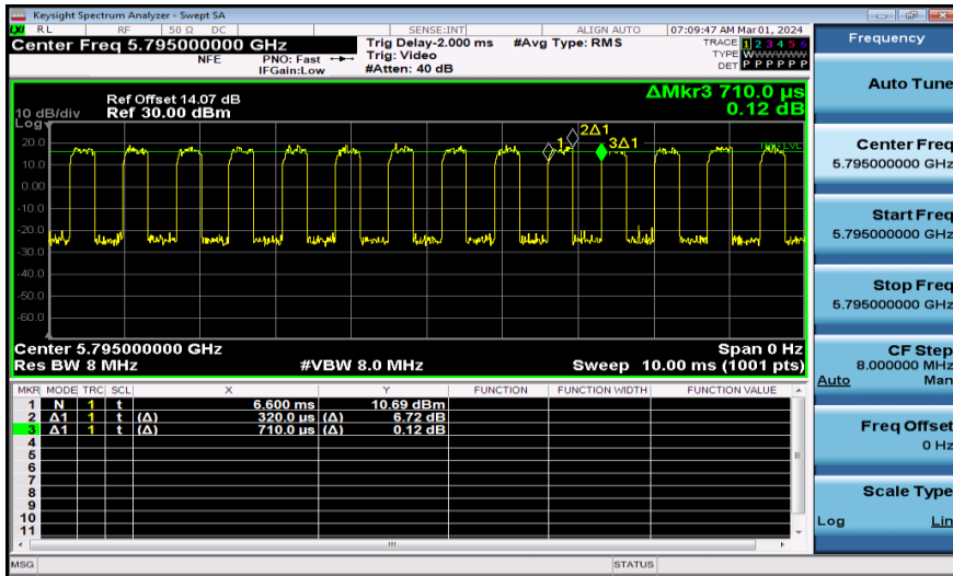
NTNV-11AX40MIMO-Ant2-5795
