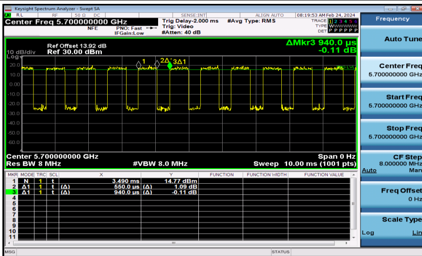
NTNV-11AX20MIMO-Ant1-5700
