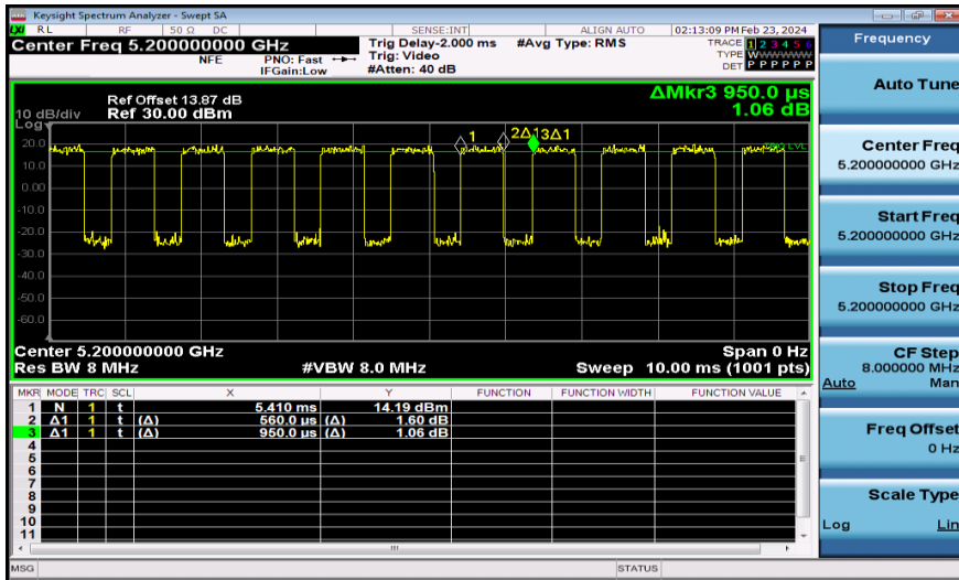
NTNV-11AX20MIMO-Ant1-5200
