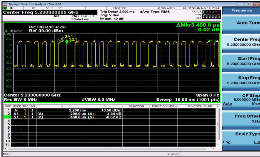
NTNV-11AX40MIMO-Ant1-5230
