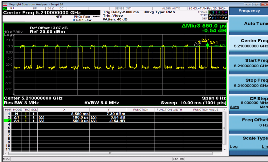
NTNV-11AC80MIMO-Ant1-5210
