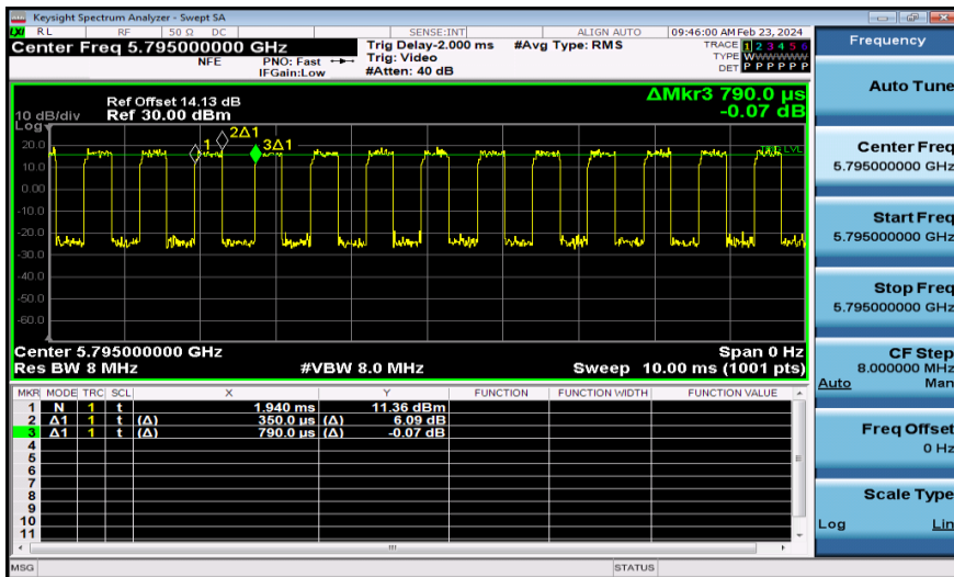
NTNV-11AC40MIMO-Ant1-5795
