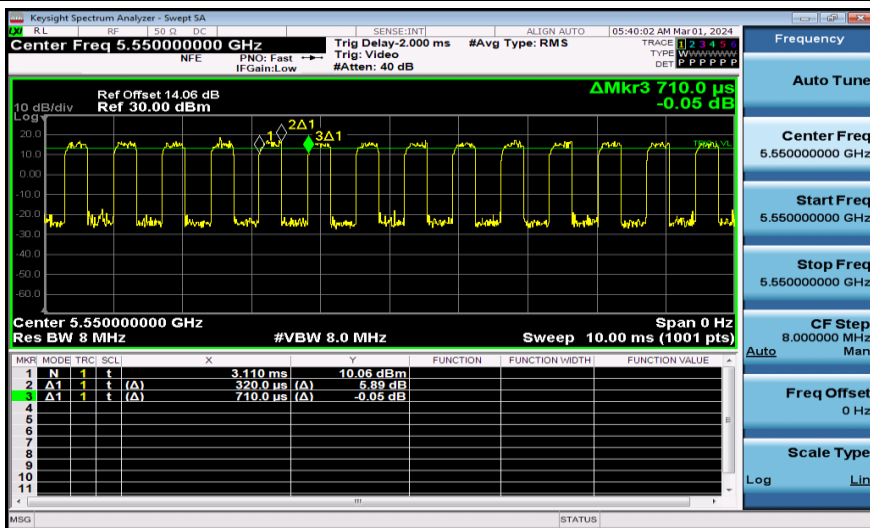
NTNV-11AX40MIMO-Ant1-5550
