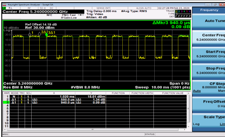
NTNV-11AX20MIMO-Ant1-5240
