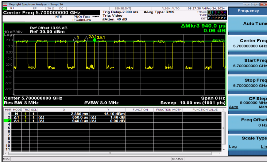
NTNV-11AX20MIMO-Ant2-5700
