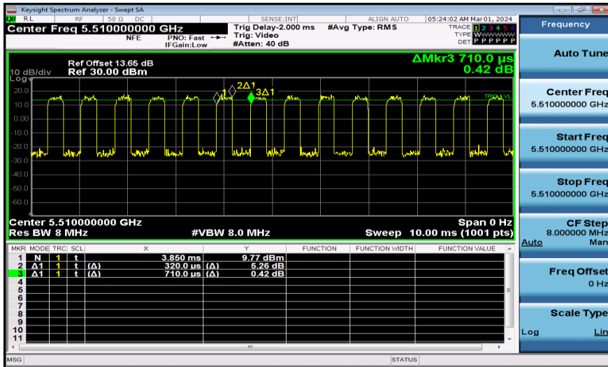
NTNV-11AX40MIMO-Ant1-5510
