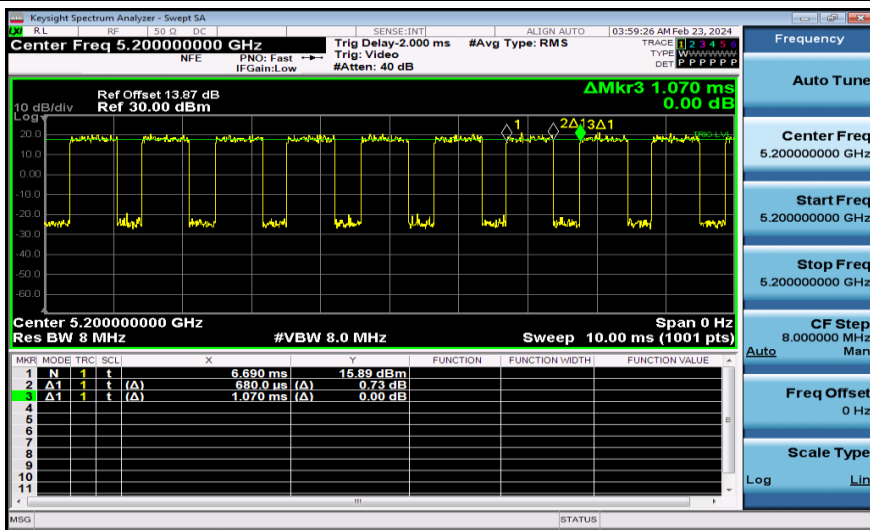
NTNV-11AC20MIMO-Ant1-5200
