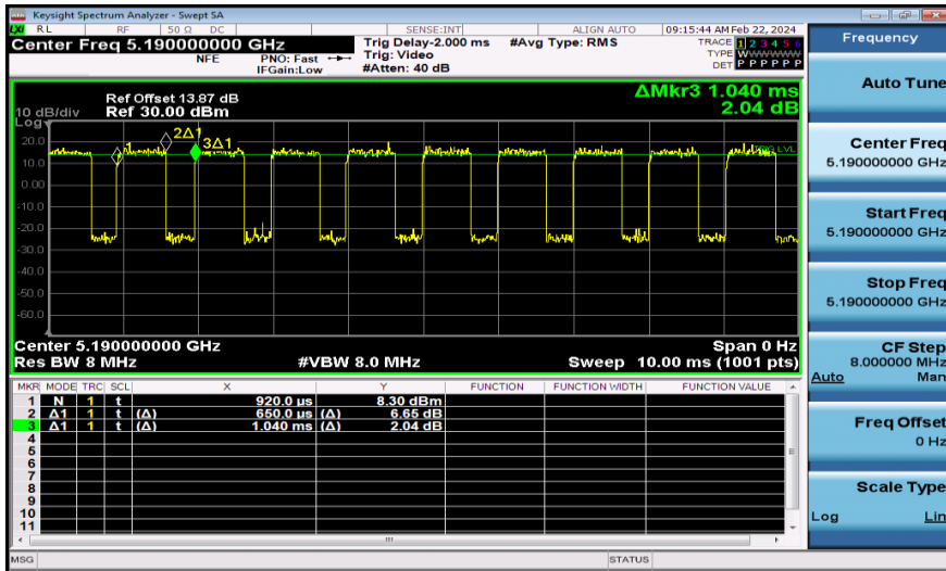
NTNV-11N40MIMO-Ant1-5190
