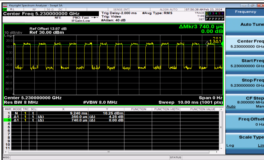
NTNV-11AC40MIMO-Ant1-5230
