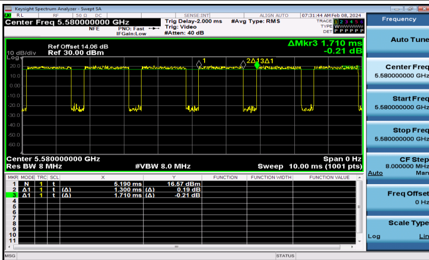
NTNV-11N20MIMO-Ant1-5580
