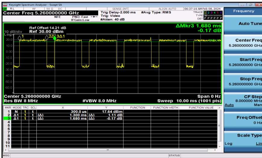
NTNV-11N20MIMO-Ant2-5260
