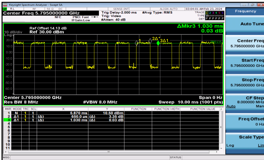
NTNV-11N40MIMO-Ant1-5795
