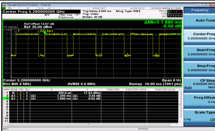
NTNV-11N20MIMO-Ant1-5200
