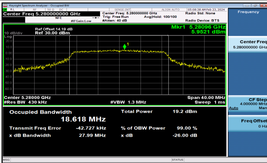
11AC20MIMO-Ant1-5280
