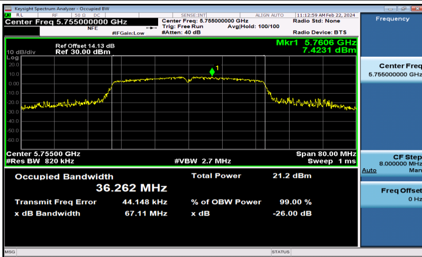
11N40MIMO-Ant1-5755
