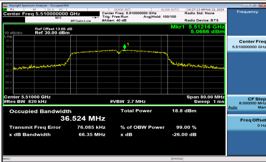
11N40MIMO-Ant1-5510
