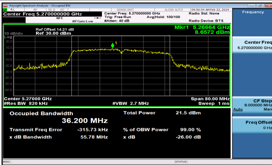
11N40MIMO-Ant2-5270
