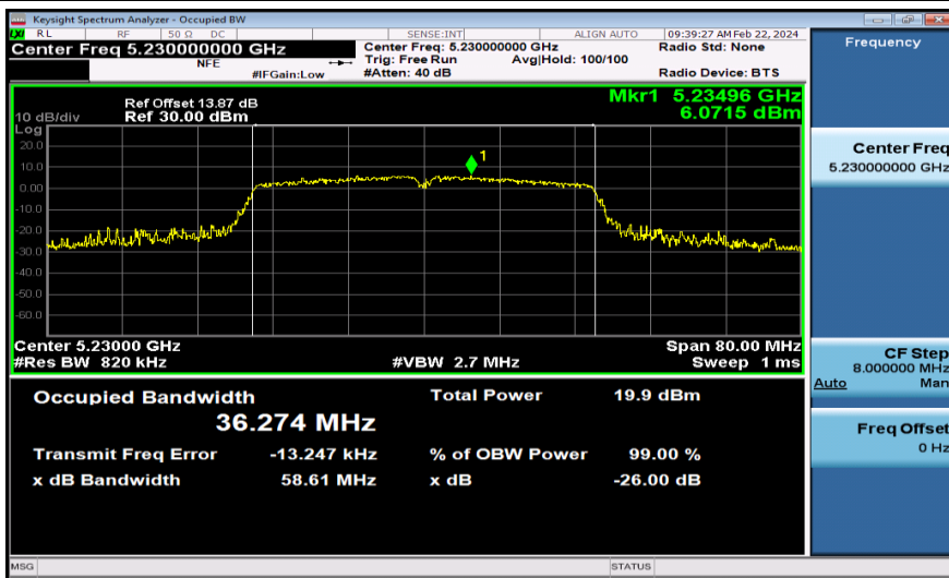
11N40MIMO-Ant1-5230
