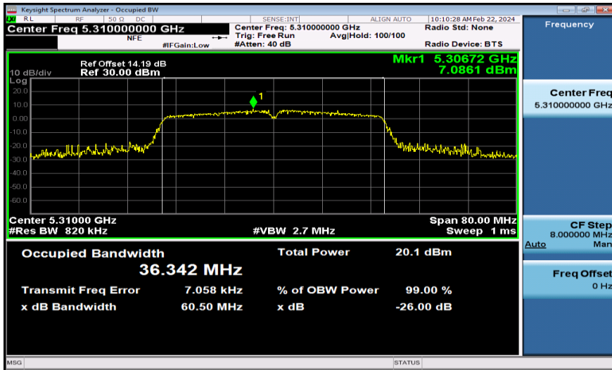
11N40MIMO-Ant1-5310
