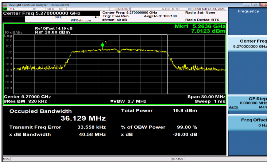
11AC40MIMO-Ant1-5270
