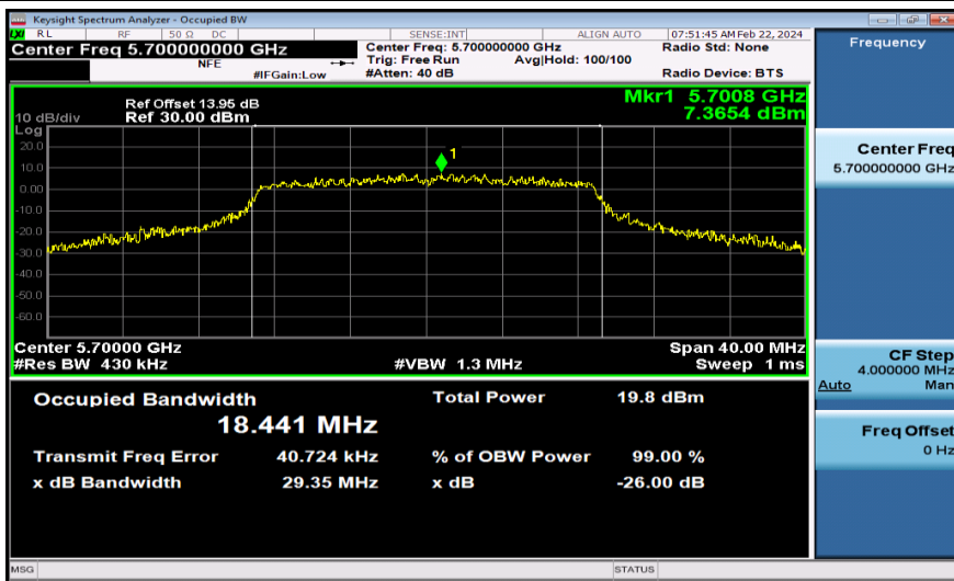
11N20MIMO-Ant2-5700
