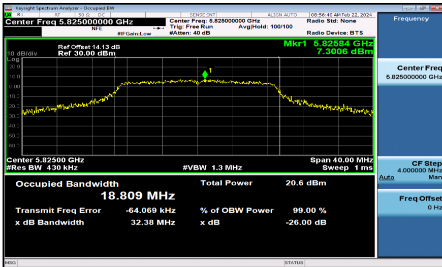
11N20MIMO-Ant1-5825
