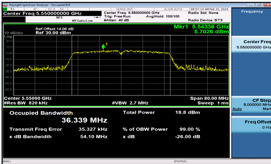
11AC40MIMO-Ant1-5550
