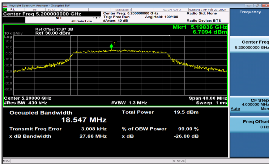
11AC20MIMO-Ant1-5200
