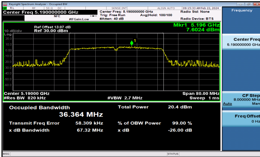
11N40MIMO-Ant1-5190
