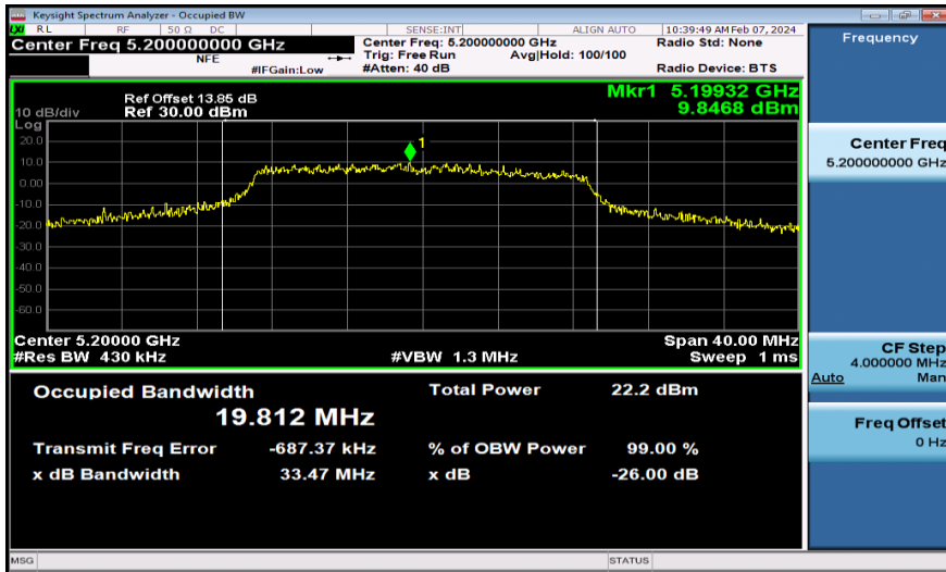
11N20MIMO-Ant2-5200
