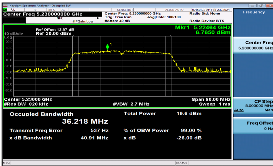
11AC40MIMO-Ant1-5230
