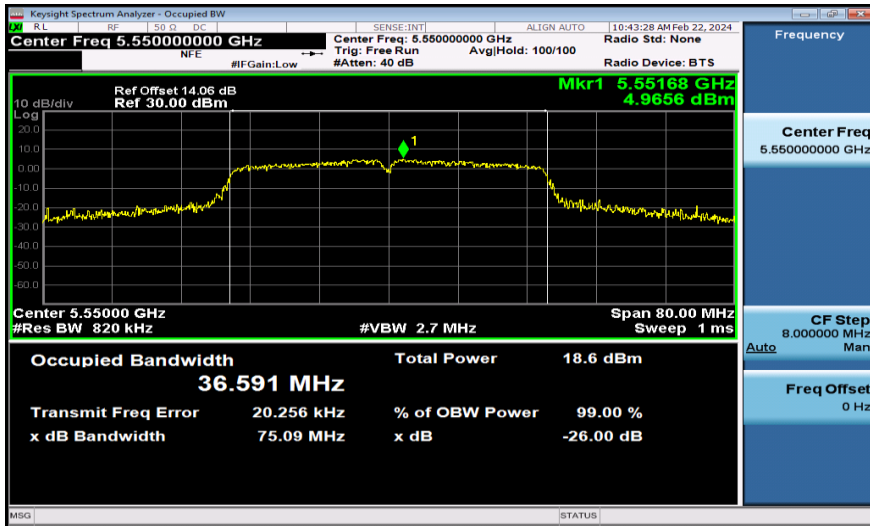
11N40MIMO-Ant1-5550
