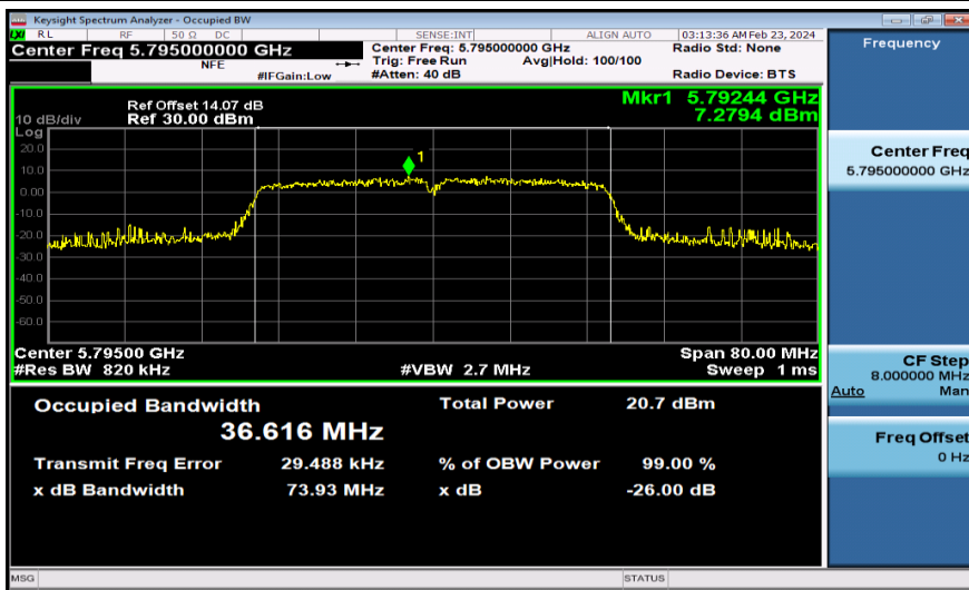
11N40MIMO-Ant2-5795
