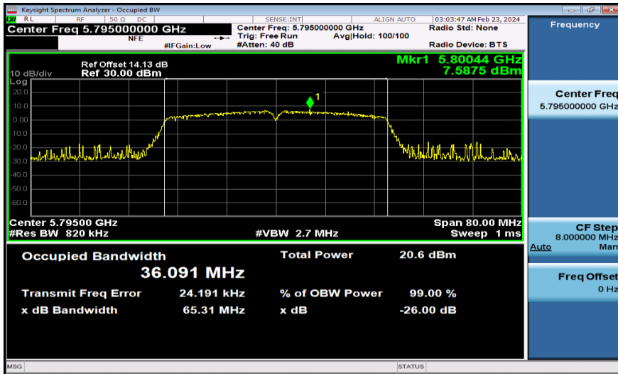
11N40MIMO-Ant1-5795
