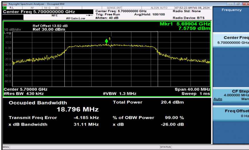
11N20MIMO-Ant1-5700
