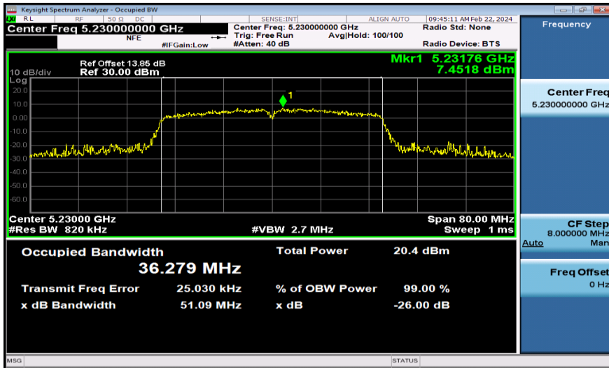
11N40MIMO-Ant2-5230
