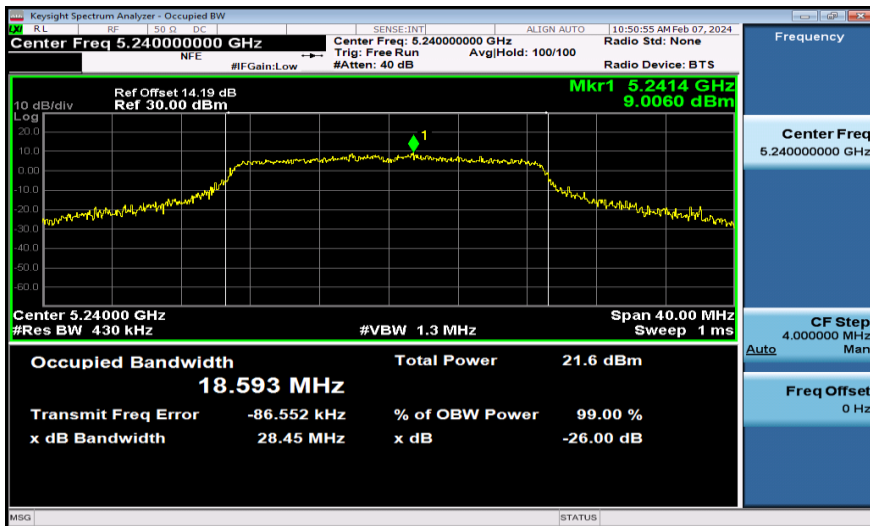
11N20MIMO-Ant1-5240
