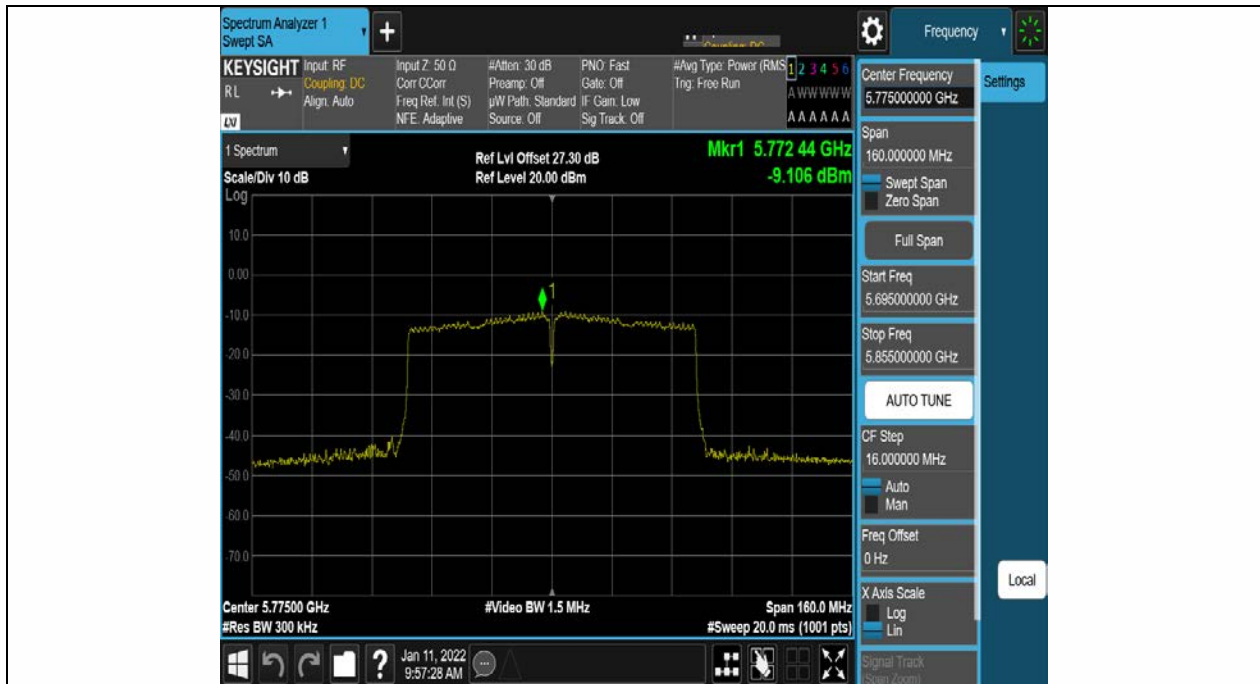
11AC80SISO_Ant1_5775
