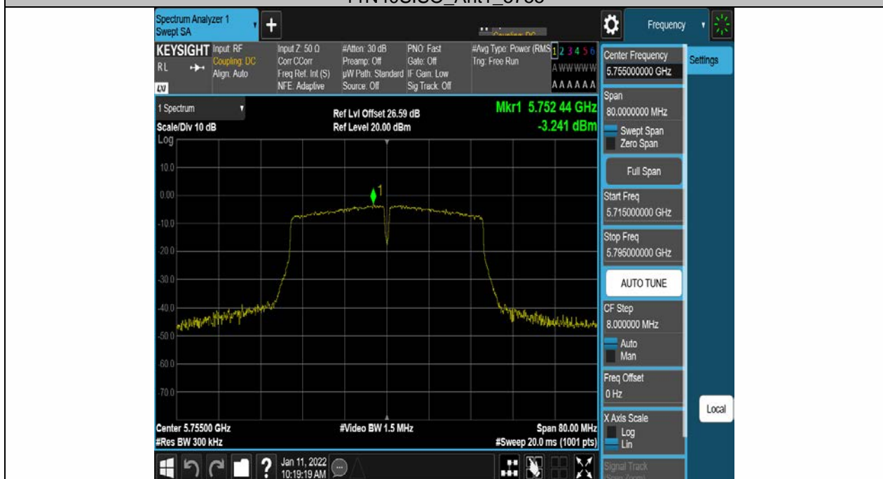
11N40SISO_Ant2_5755
