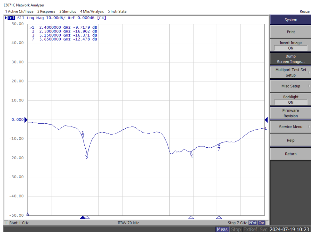
S-parameter
