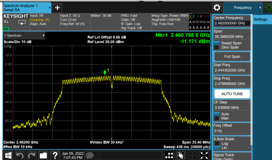
11N20MIMO Ant1 2462
