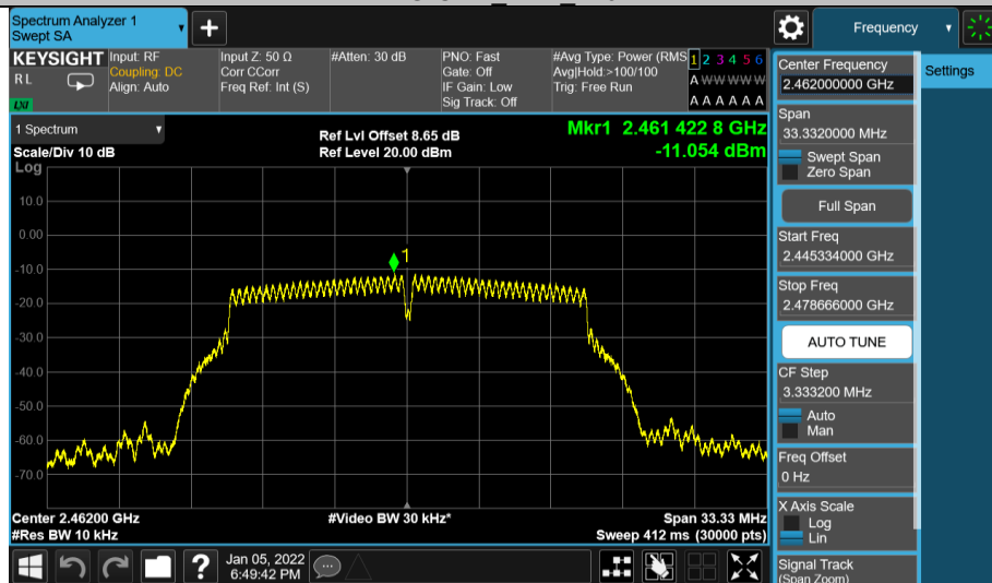
11G-CDD Ant1 2462
