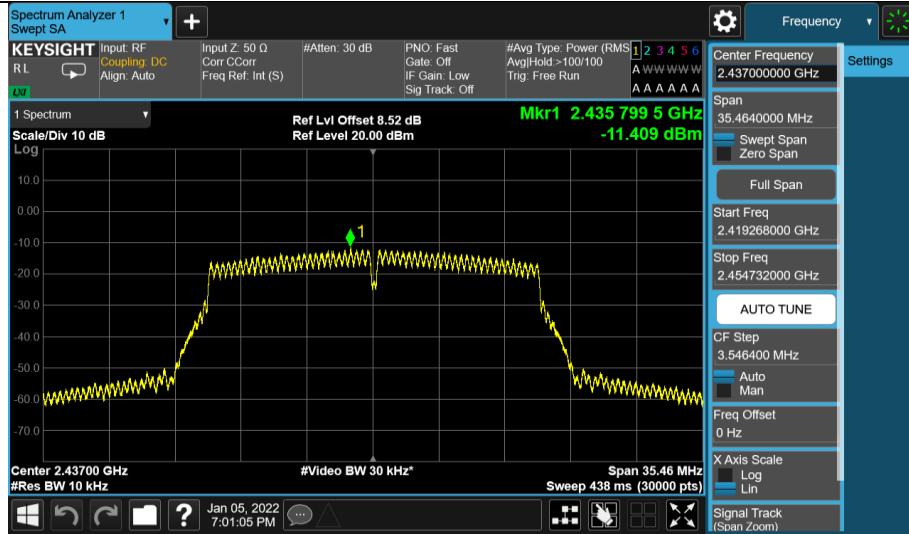
11N20MIMO Ant2 2437
