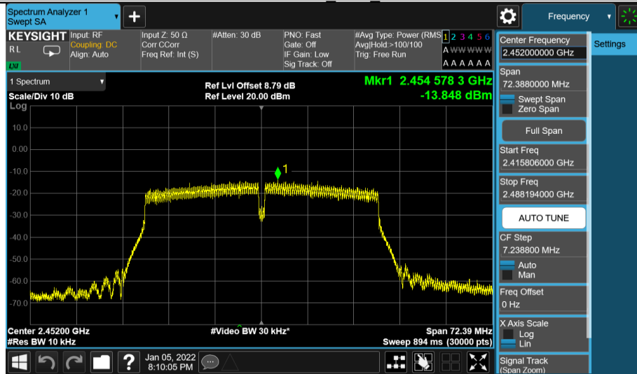
11N40MIMO Ant1 2452
