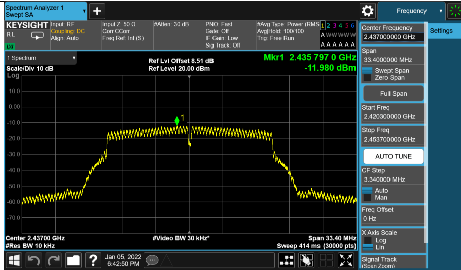
11G-CDD Ant2 2437
