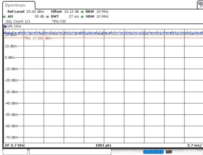
11N20SISO_Ant2_5700
