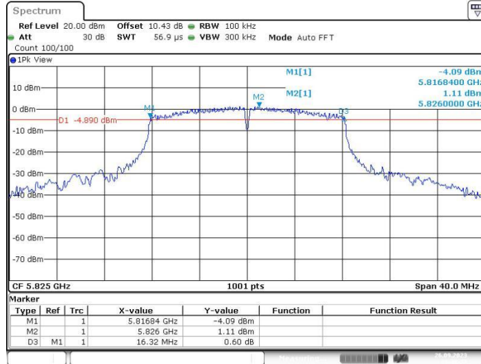
11A_Ant2_5825
