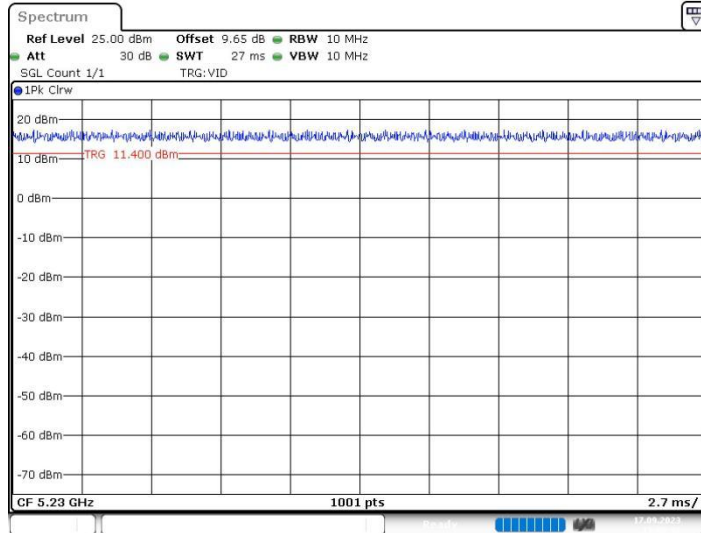
11N40SISO_Ant2_5230
