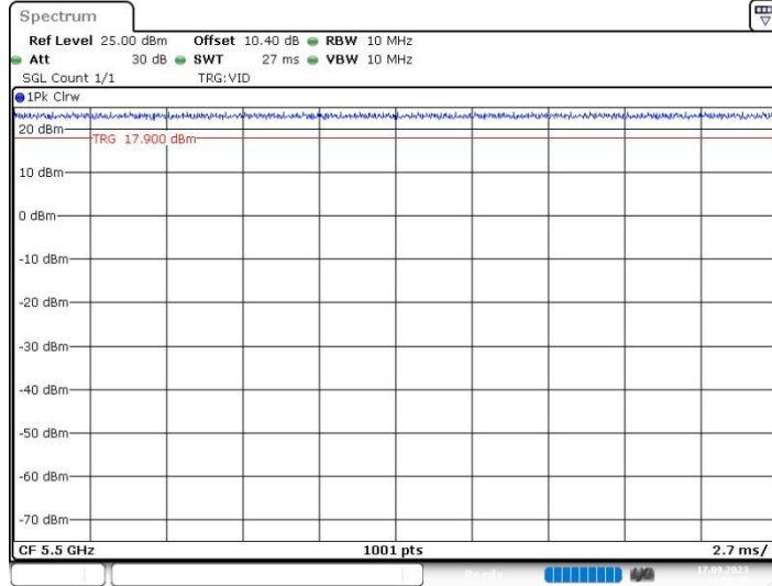
11N20SISO_Ant2_5500
