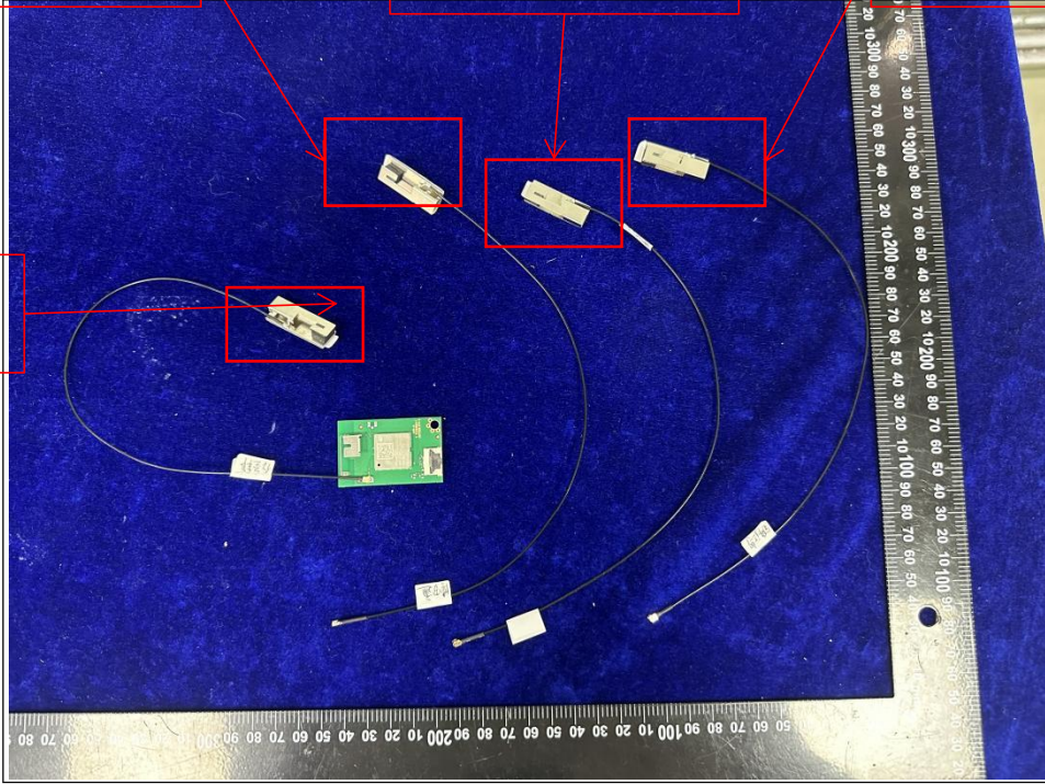
Antenna1 1# TX-DM200BD113B63
