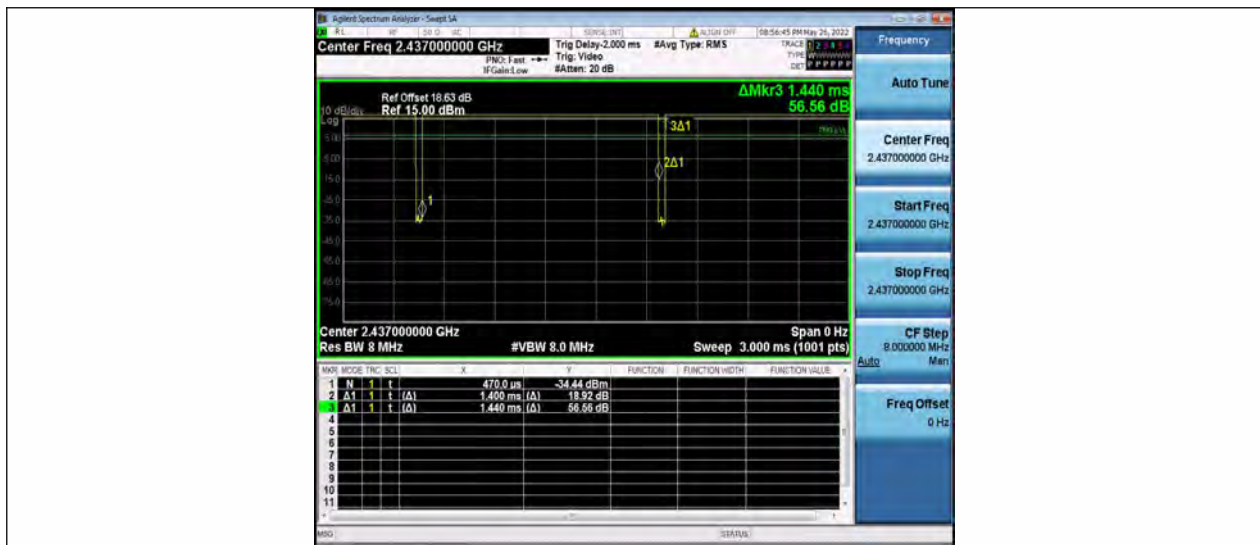
11G_Ant2_2437
