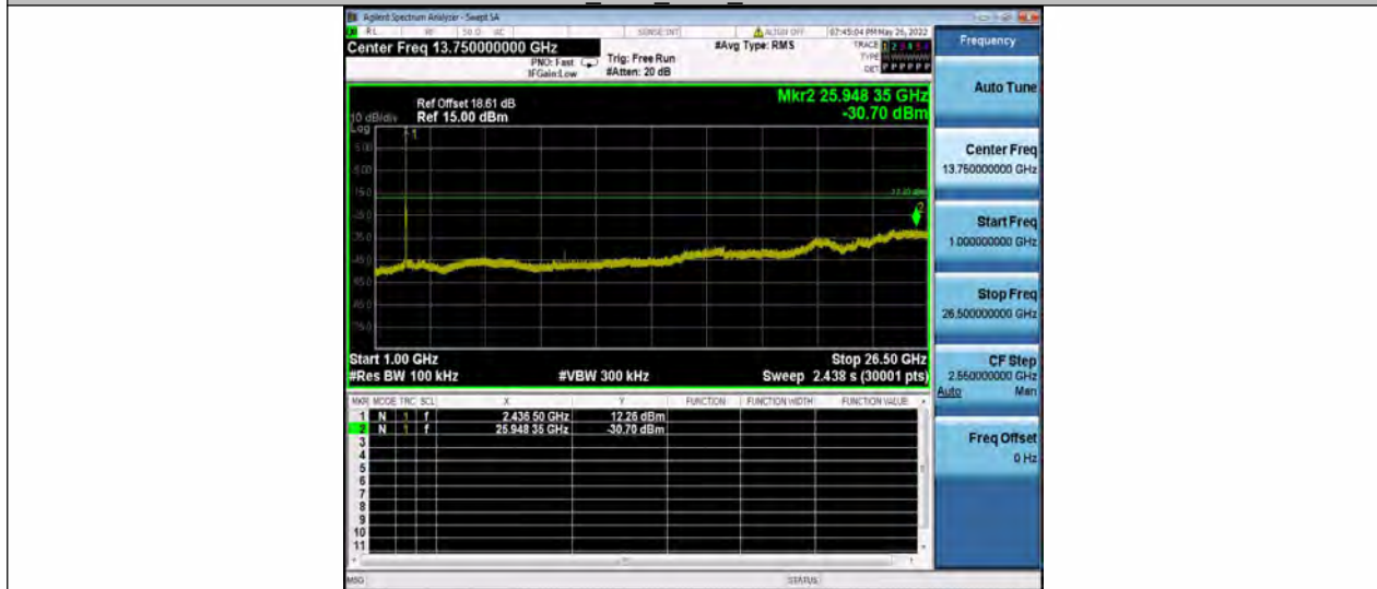
11B_Ant1_2437_1000~26500
