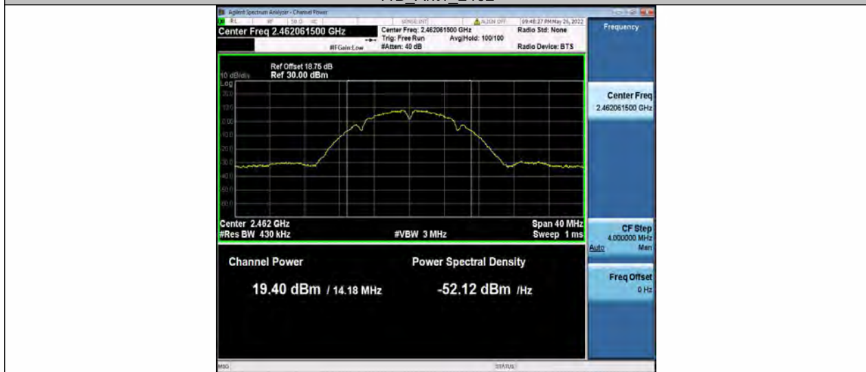
11B_Ant2_2462
