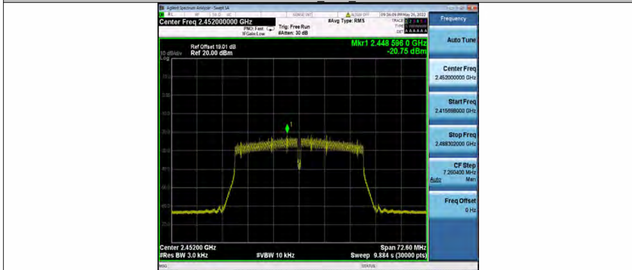
11N40SISO_Ant2_2452
