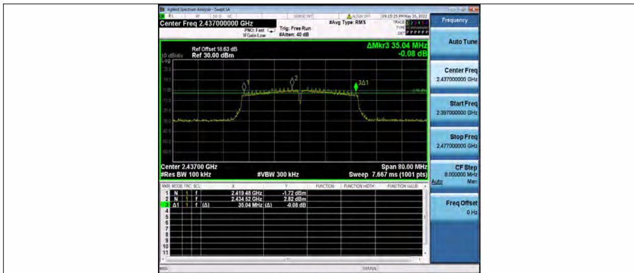
11N40SISO_Ant2_2437
