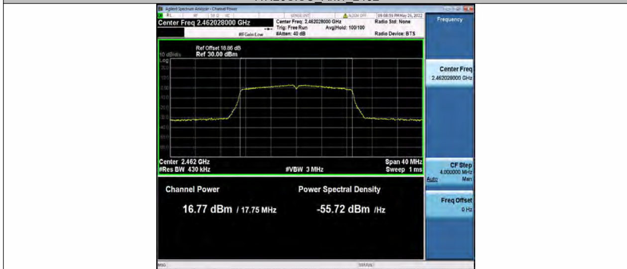
11N20SISO_Ant2_2462
