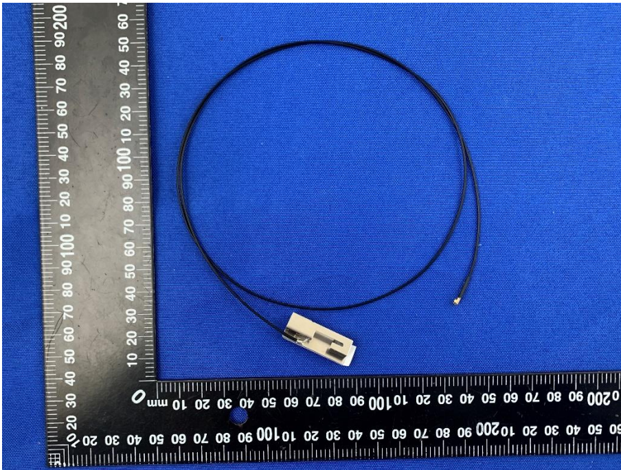
PIFA ANTENNA-735mm
