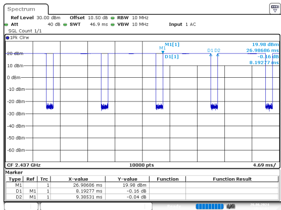
b_2437MHz_Chain 0
