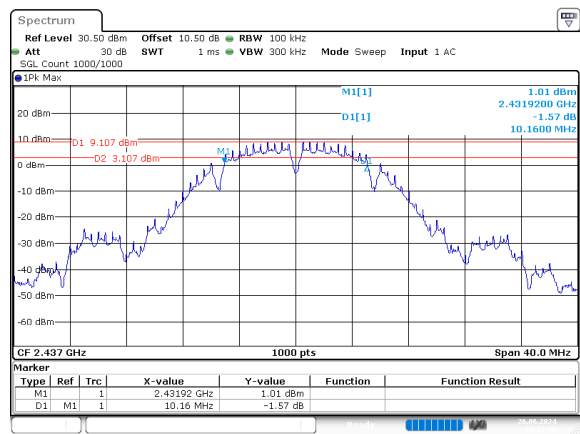
b_2437MHz_Chain 0
