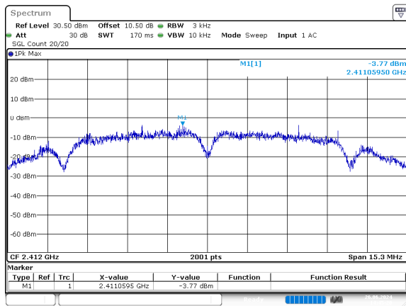
b_2412MHz_Chain 0
