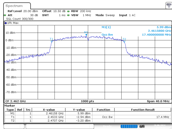
n20_2462MHz_Chain 0
