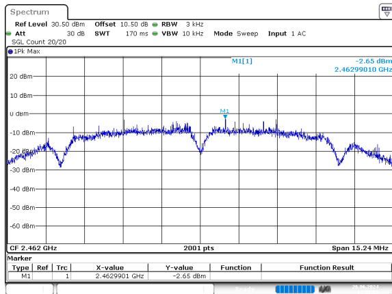
b_2462MHz_Chain 0
