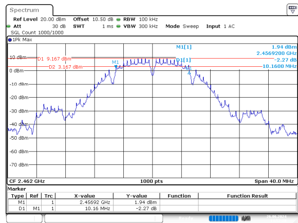
b_2462MHz_Chain 0
