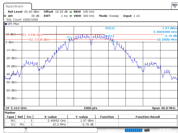
b_2412MHz_Chain 0
