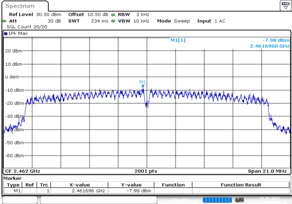
n20_2462MHz_Chain 0
