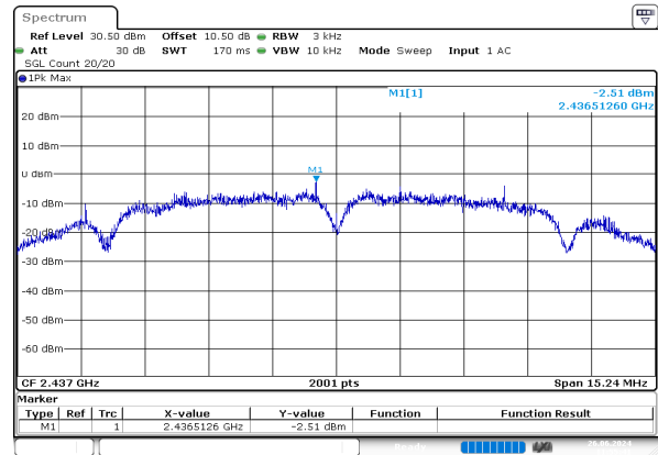
b_2437MHz_Chain 0
