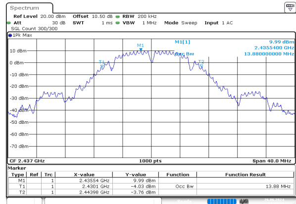
b_2437MHz_Chain 0
