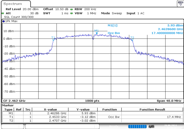
n20_2462MHz_Chain 0
