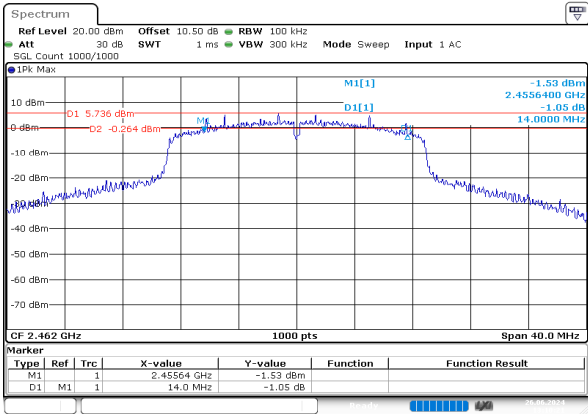
n20_2462MHz_Chain 0
