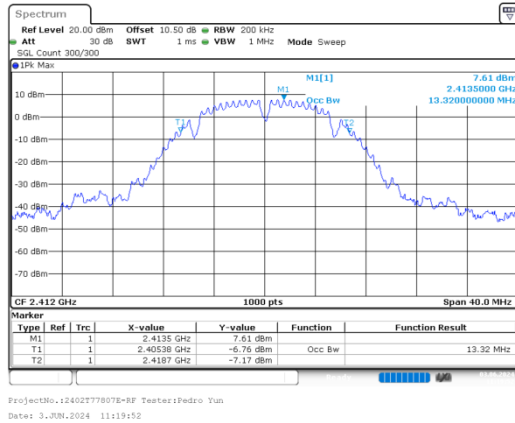
b_2412MHz_Chain 0
