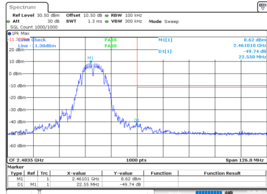
b_2462MHz_Chain 0
