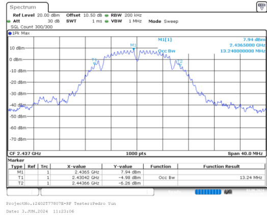
b_2437MHz_Chain 0
