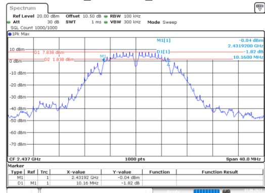
b_2437MHz_Chain 0
