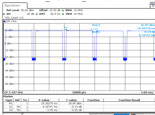
b_2437MHz_Chain 0
