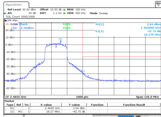
n20_2462MHz_Chain 0
