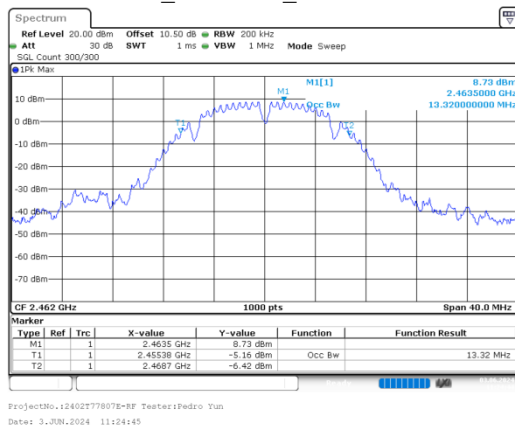
b_2462MHz_Chain 0
