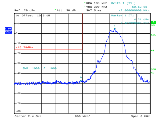
BLE 1Mbps Low
