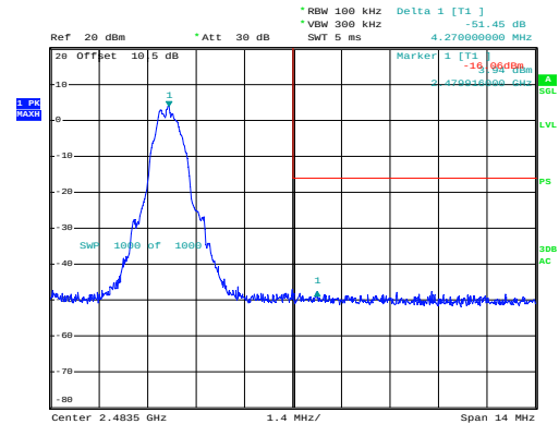
BLE 1Mbps High
