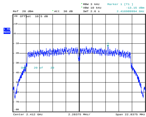
n20_2412MHz_Chain 1
