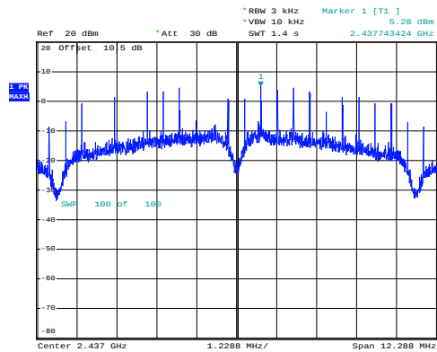
b_2437MHz_Chain 0
