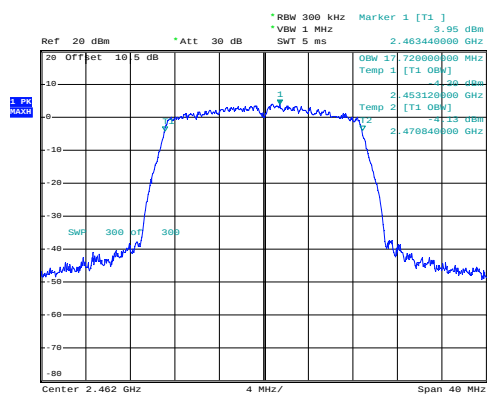
n20_2462MHz_Chain 0
