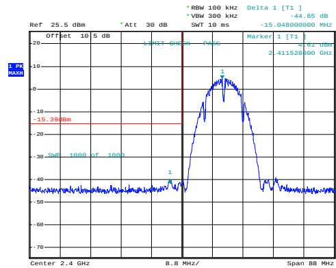
b_2412MHz_Chain 1
