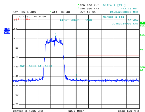
n20_2462MHz_Chain 1
