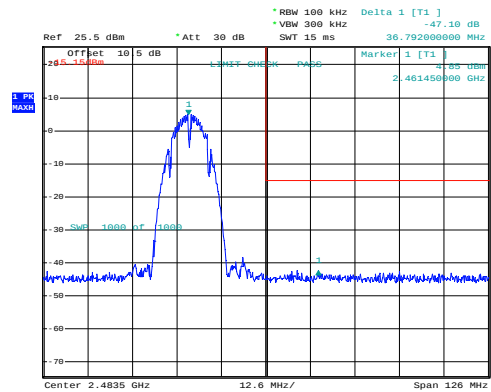
b_2462MHz_Chain 1
