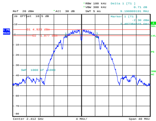
b_2412MHz_Chain 0
