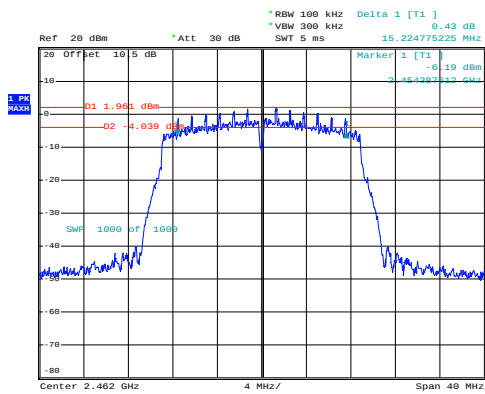
n20_2462MHz_Chain 0
