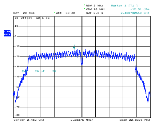
n20_2462MHz_Chain 1
