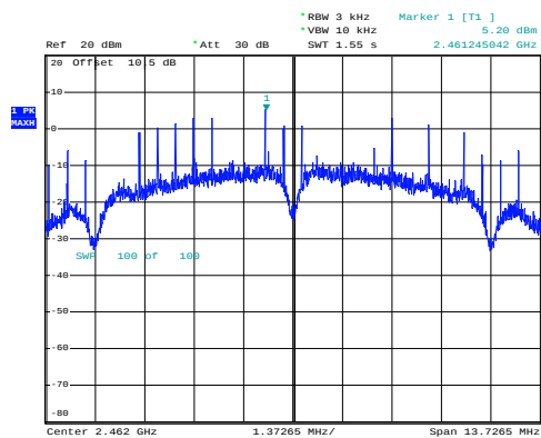
b_2462MHz_Chain 0
