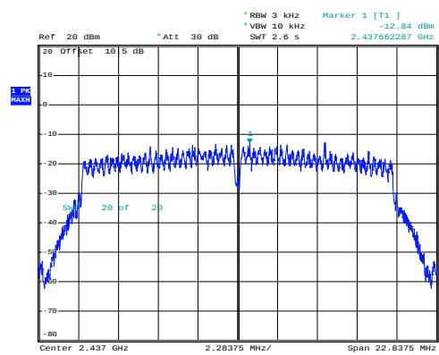
n20_2437MHz_Chain 1
