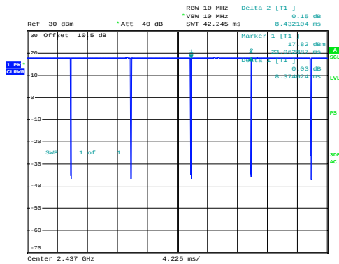
b_2437MHz_Chain 0
