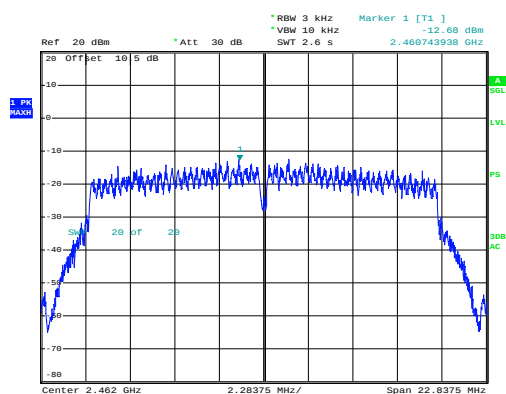
n20_2462MHz_Chain 0
