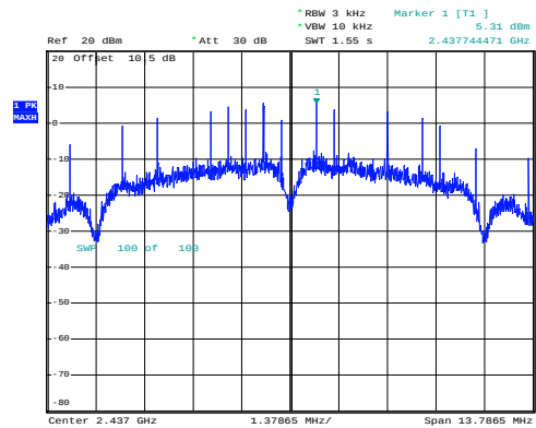
b_2437MHz_Chain 1
