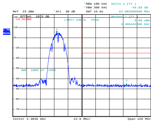
b_2462MHz_Chain 0
