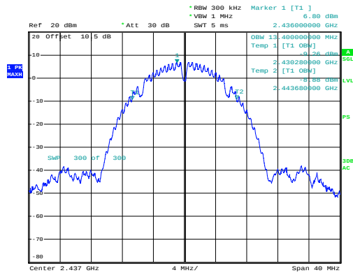
b_2437MHz_Chain 0
