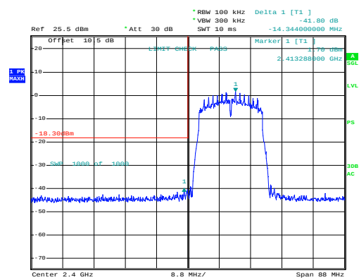
n20_2412MHz_Chain 1
