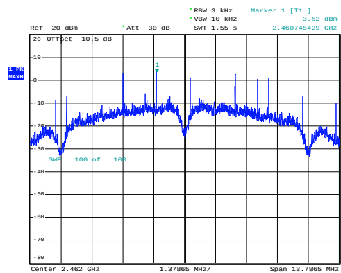
b_2462MHz_Chain 1
