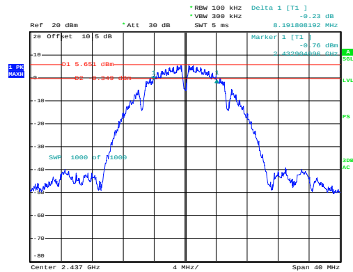
b_2437MHz_Chain 0
